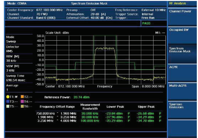
CDMA ACPR
