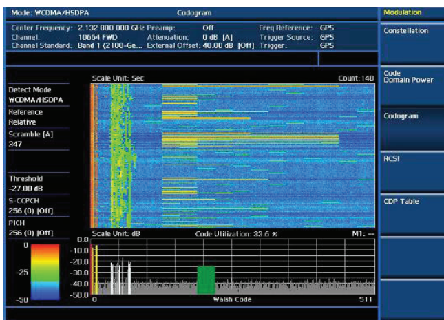
WCDMA codogram
