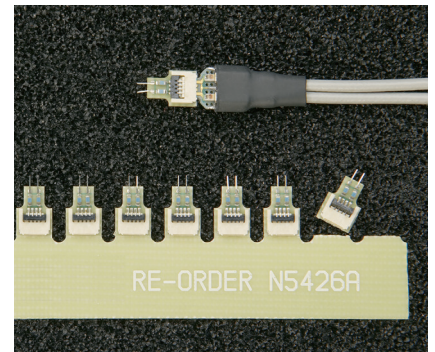
Figure 13. New InfiniiMax ZIF probe head (N5425A) and ZIF tips (N5426A) for your DDR2 probing solution.
