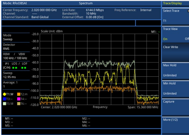
RfOBSAI – Spectrum
