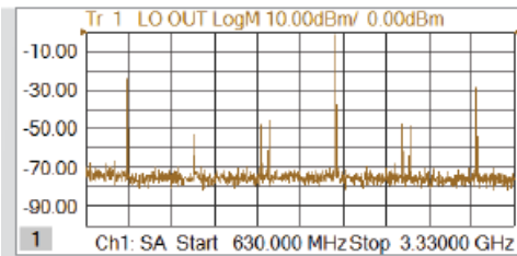
Output spectrum on LO port
