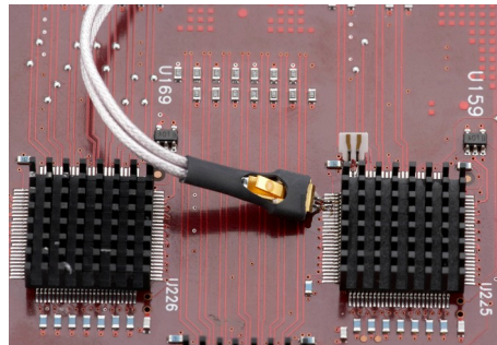
InfiniiMax III ZIF head and tip
