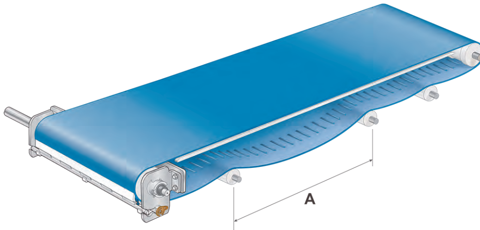
図 71: 正しいサポートの間隔
