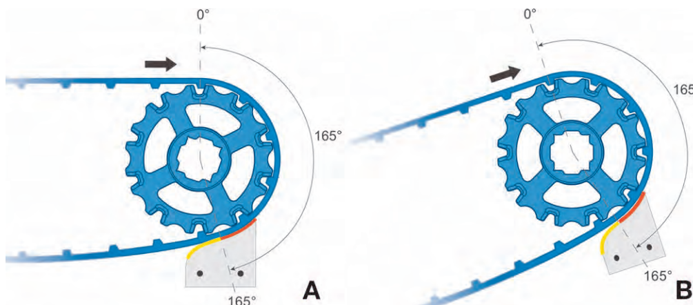
図 56: 先頭駆動のポジションリミターの配置
