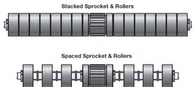
図 6: S8240 シングルレ恩斯プロケット/ローラー/スペーサー
