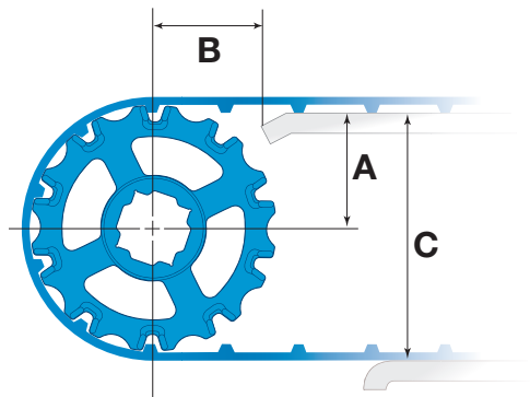
図 14: 駆動側寸法
