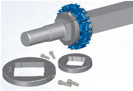
図 16: 分割重荷重用固定リング
