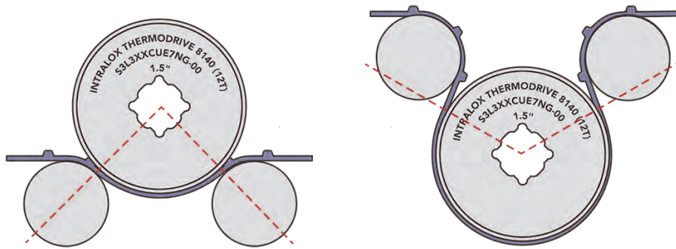
図 74: 90 度および 225 度のベルトとスプロケットの噛み合い
