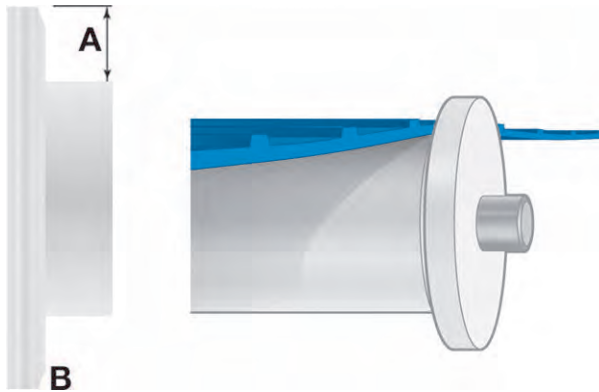
図 64: 最小クリアランスと必要な面取り
