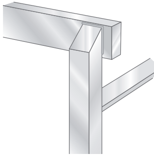
図 31: 正しいジョイントアセンブリ
