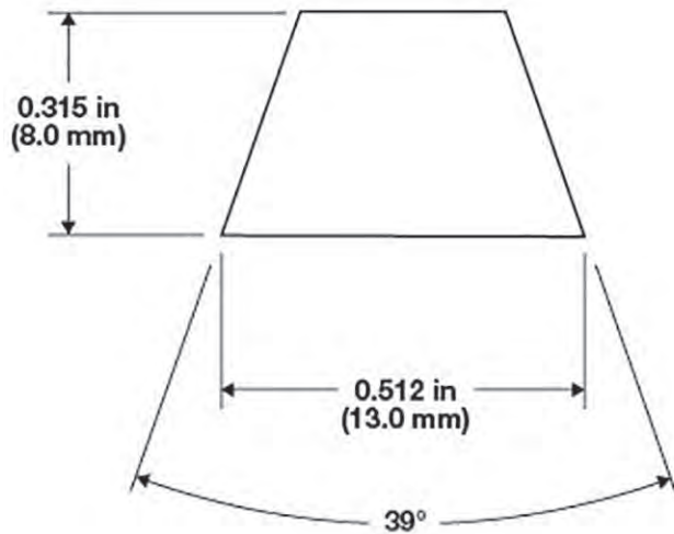
図 11: V ガイドの公称形状
