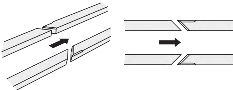
図 68: 45°角に面取りされたレール
