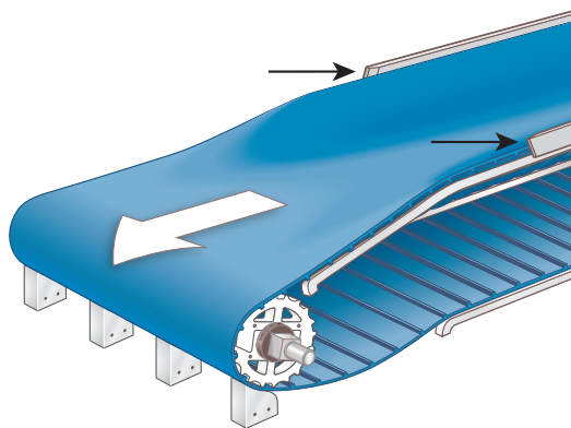
図 81: UHME-PE 製の保持レール
