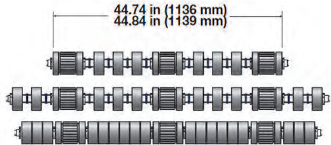
図 8: S8240 トリプルレーンспロケット/ローラー/スパーサー
