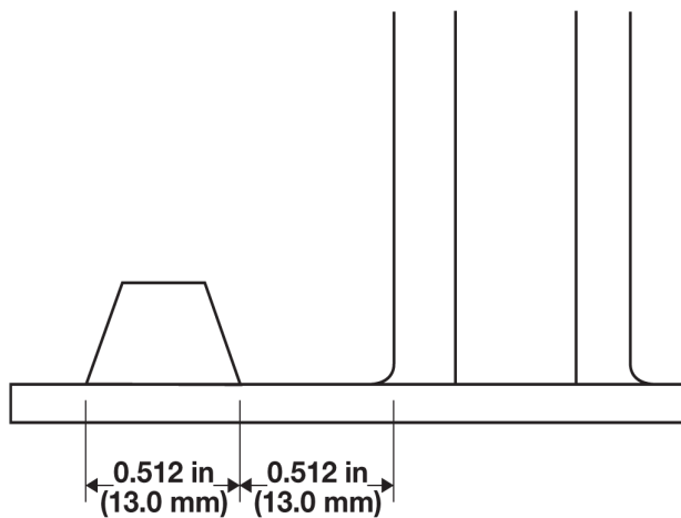
図 12: V ガイド 1 レーン分のインデント
