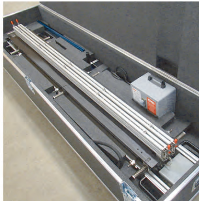
図 23: ThermoDrive®ストリームライン接合セットとコンポーネント
