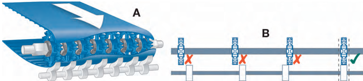
図 55: 付属品なしのベルトの正しい位置決めと最小クリアランス
