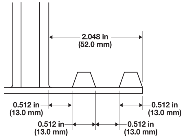
図 13: V ガイド 2 レーン分のインデント
