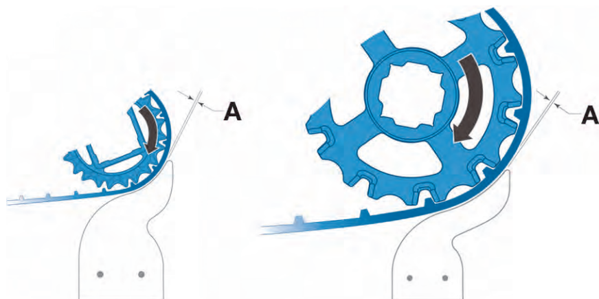
A 0.005~0.05 インチ (0.13~1.25 mm) の間隔
