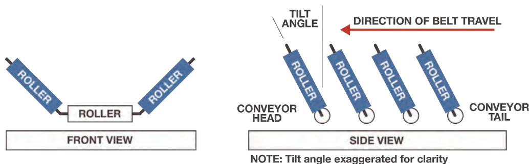
図 69: ベルト進行方向と傾斜角
