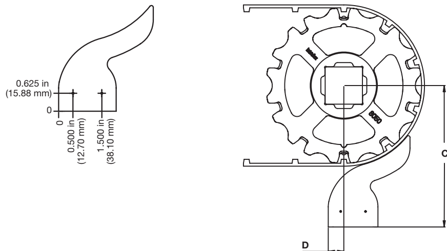
ポジションリミターブロックのデータ
