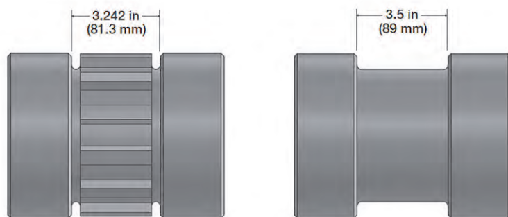
図 76: スプロケットとローラー内側寸法
