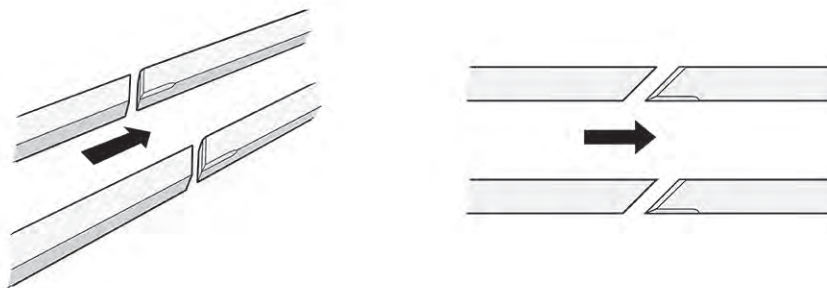
図 34: 45°角に面取りされたレール
