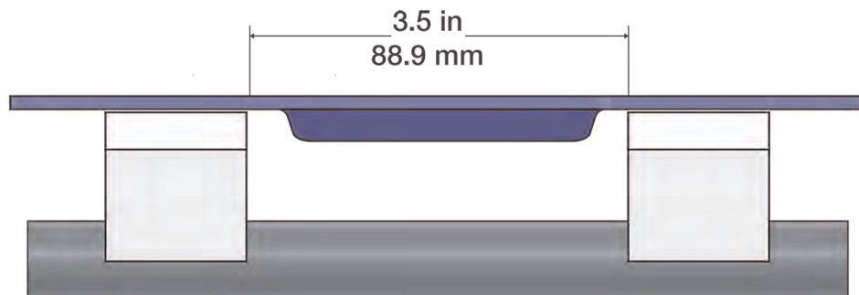
図 77: 保持レール間のシングルラグ
