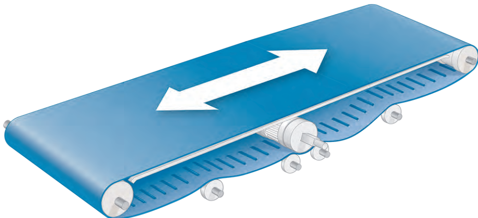
図 73: センター駆動スプロケットとポジションリミターの位置
