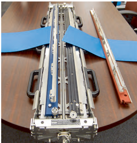
図 22: ThermoDrive 接合システム V2 およびコンポーネント
