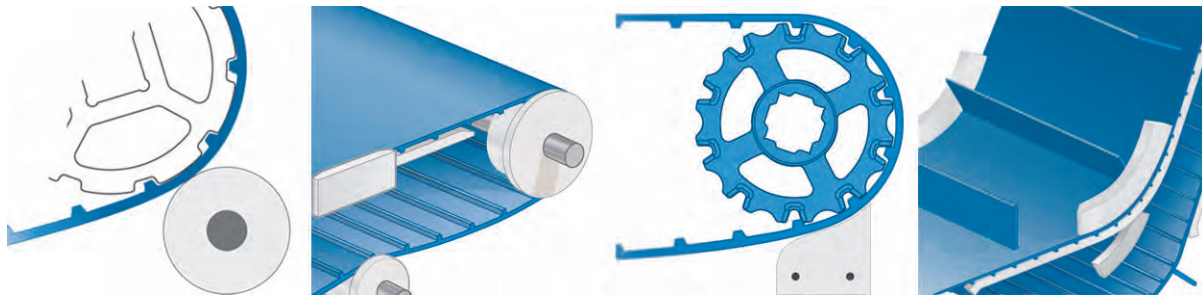
図 27: 最小曲げ半径以上のコンポーネント
