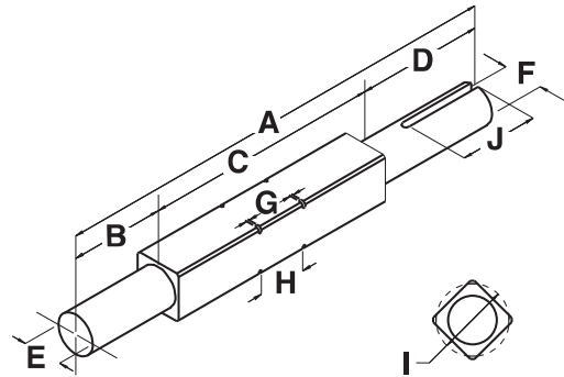
図 15: シャフトコンポーネント
