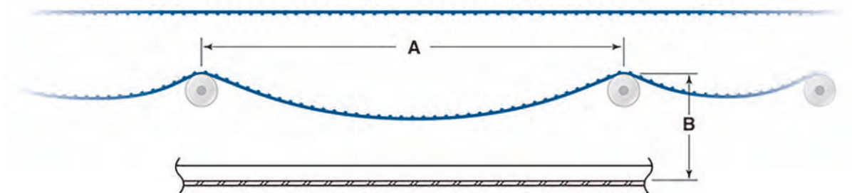
図 41: 懸垂たるみ
