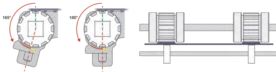
図 75: ポジションリミターの 165°～180°での配置
