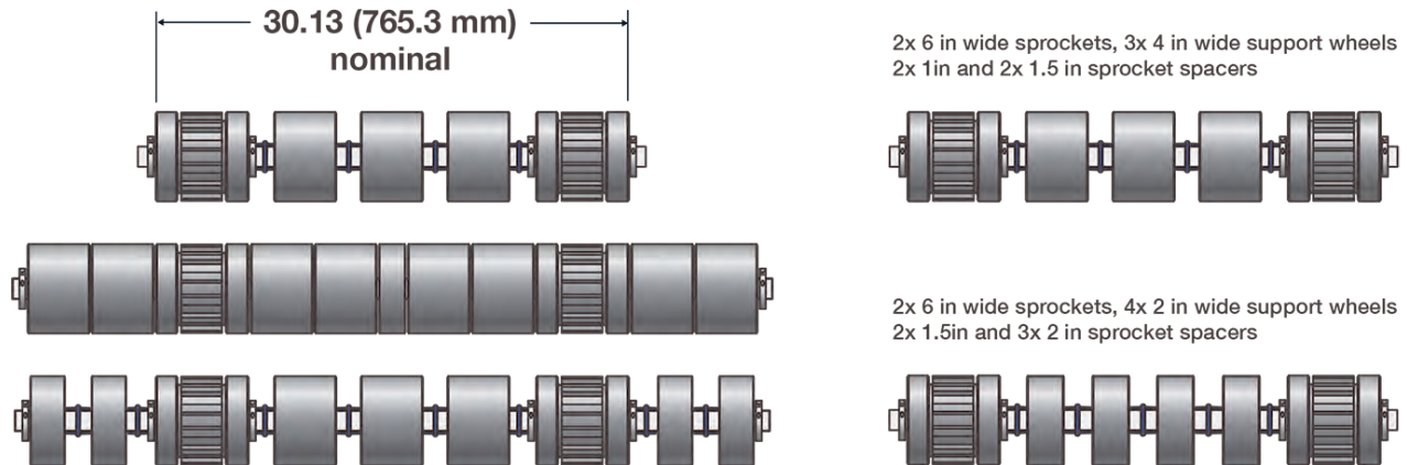
図 3: 駆動スプロケットと従動シャフトの配置間隔
