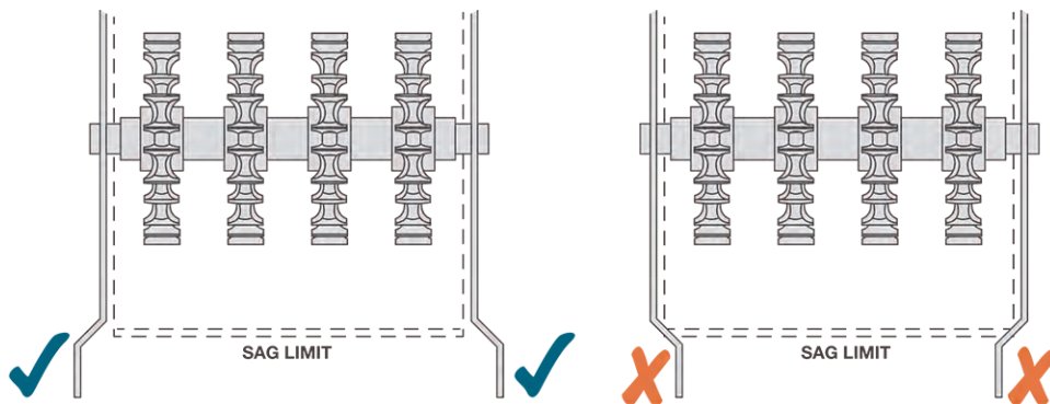
図 42: 正しいクリアランス
