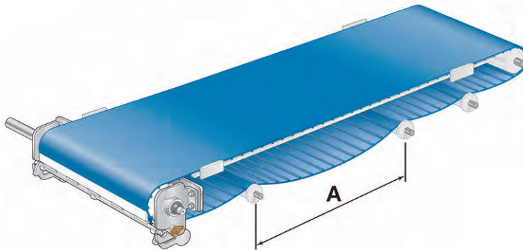
図 44: 正しいサポートの間隔
