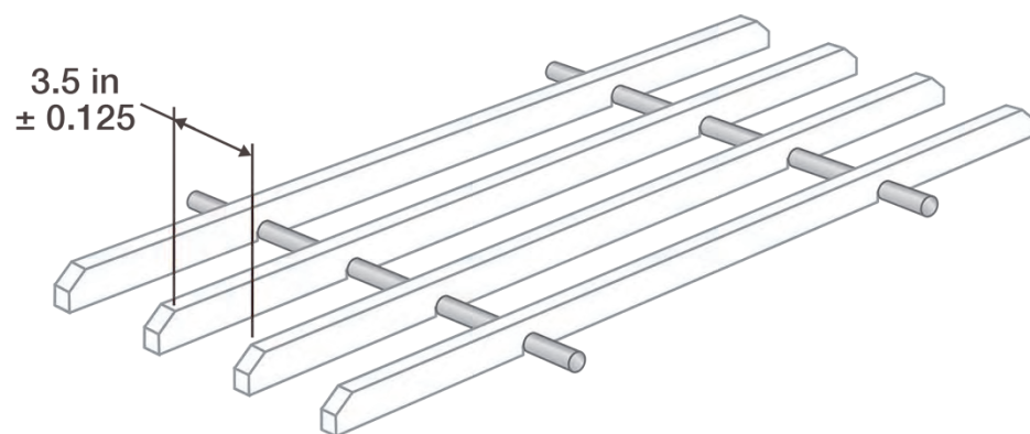
図 78: 保持レール間の隙間の寸法
