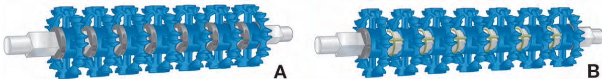
図 50: 固定リングとスプロケットスペーサー
