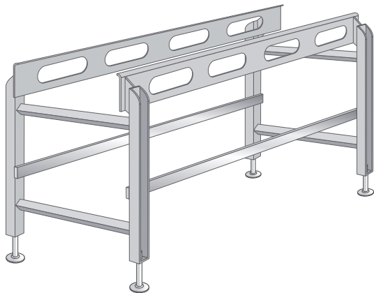
図 30: 衛生処理のためにたやすくアクセスできる簡単な構造
