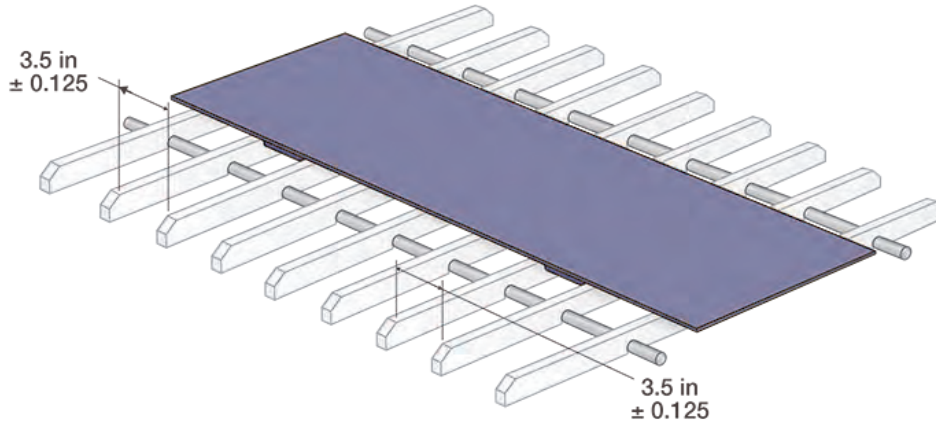
図 80: デュアルラグの隙間
