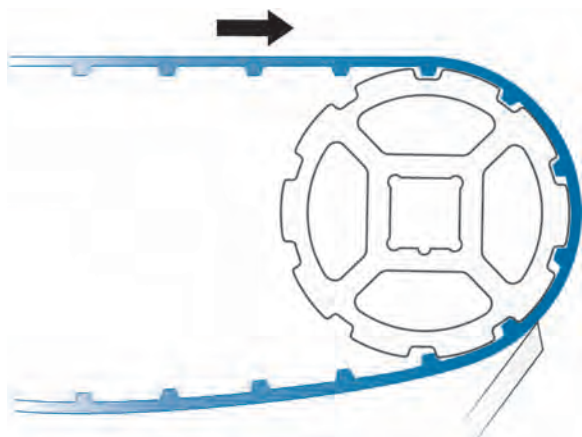
Figura 59: Raschiatore con montaggio in posizione inclinata
