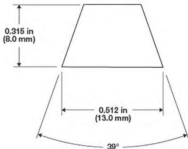
Figura 11: Geometria nominale della guida trapezoidale
