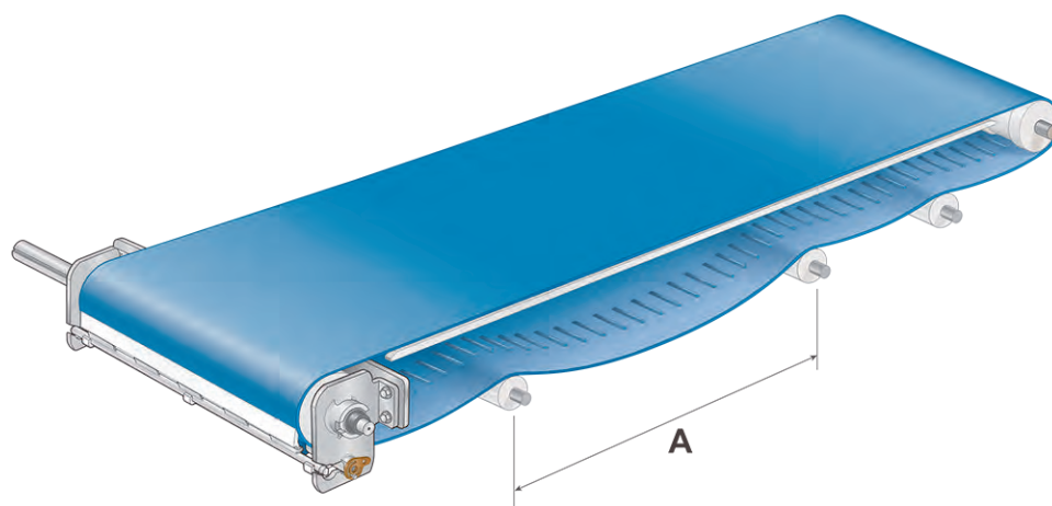
Figura 71: Corretta spaziatura del supporto
