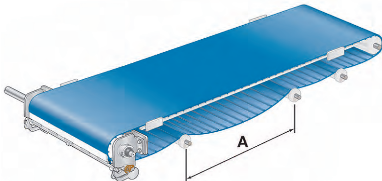
Figura 44: Corretta spaziatura del supporto
