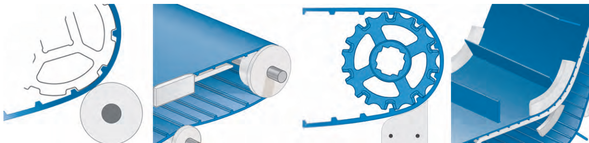
Figura 27: Componenti in corrispondenza o al di sopra del raggio di curvatura minimo
