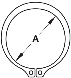
Figura 18: Diametro scanalatura anello di bloccaggio
