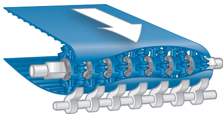
Figura 49: Installazione dei pignoni esterni
