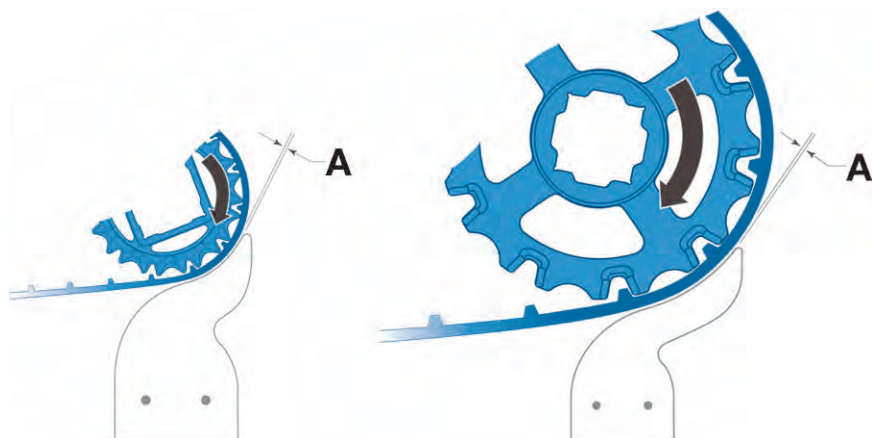
Figura 52: Corretto posizionamento del limitatore
