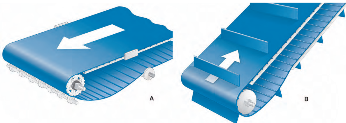
Figura 39: Accumulo del nastro
