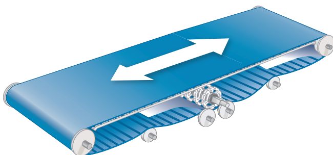
Figura 57: Posizione del pignone di azionamento centrale e del limitatore di posizione
