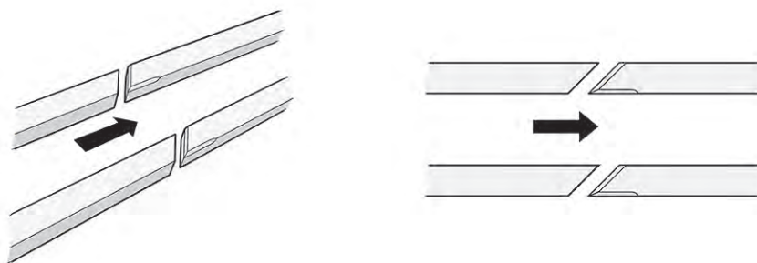
Figura 34: Guide smussate a un angolo di 45°
