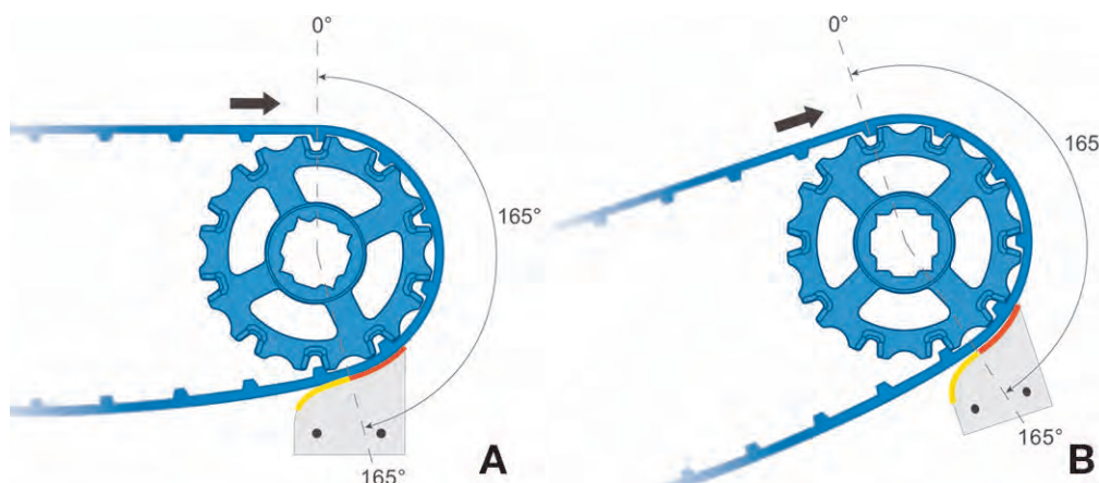
Figura 56: Posizionamento del limitatore di posizione nell'azionamento dall'estremità
