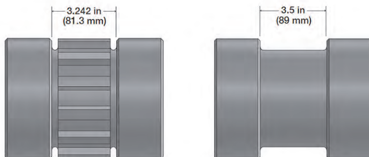
Figura 76: Dimensioni interne del pignone e del rullo
