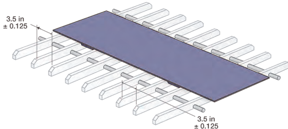
Figura 80: Spazio per doppia fila di denti
