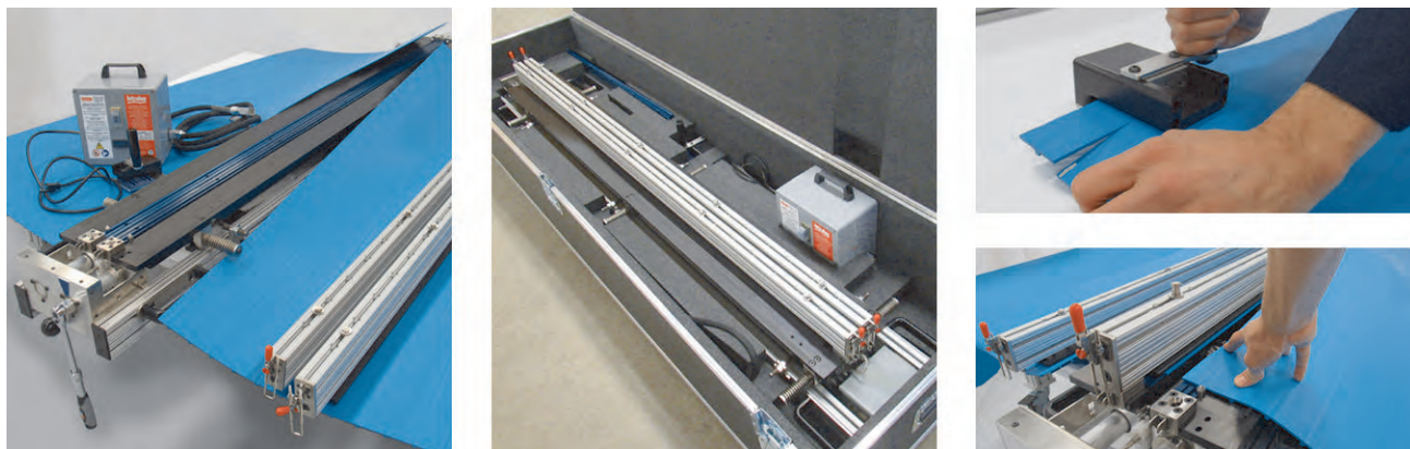
Figura 23: Sistema di giunzione ottimizzato ThermoDrive® e componenti
