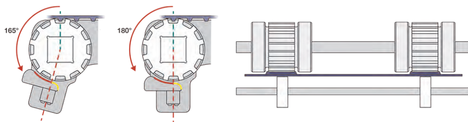
Figura 75: Posizionamento del limitatore di posizione tra 165 e 180 gradi
