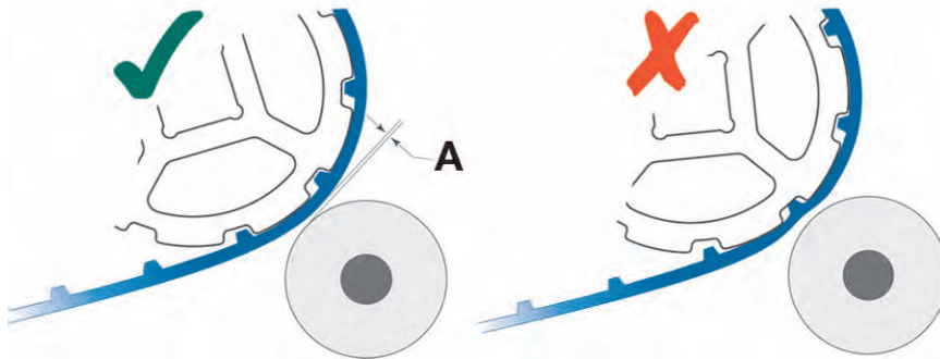
Figura 53: Posizionamento corretto del dente del pignone al di sotto del nastro durante il posizionamento del limitatore a rullo
