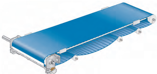
Figura 40: Sagola catenaria tra i componenti
