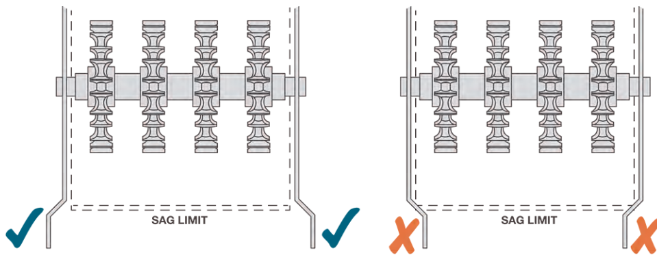
Figura 42: Gioco corretto
