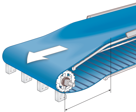
Figura 82: Corretta distanza di transizione
