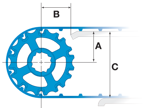
Figura 14: Dimensioni delle estremità di azionamento
