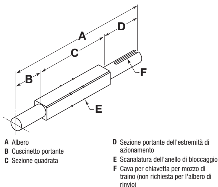
Figura 48: Componenti dell'albero motore a sezione quadra
