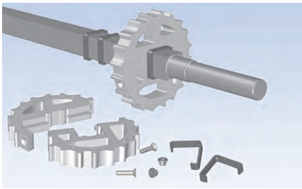
Figura 17: Anello di bloccaggio autobloccante
