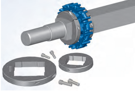
Figura 16: Anello di bloccaggio in due metà per impieghi gravosi
