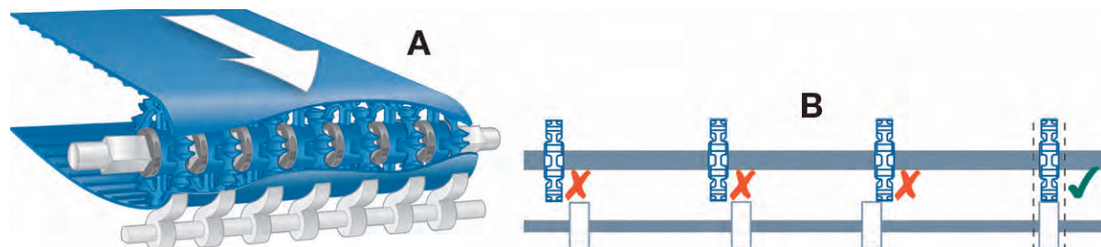
Figura 55: Allineamento e gioco minimo corretti per i nastri senza accessori
