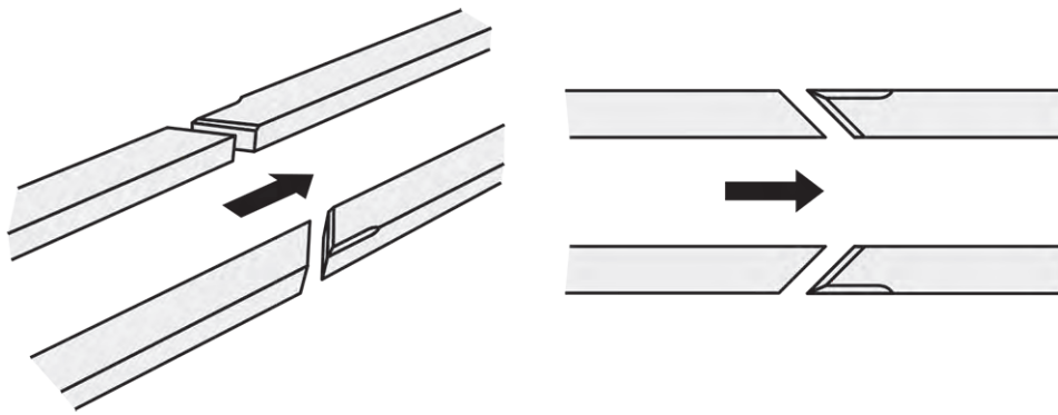
Figura 68: Guide smussate a un angolo di 45°
