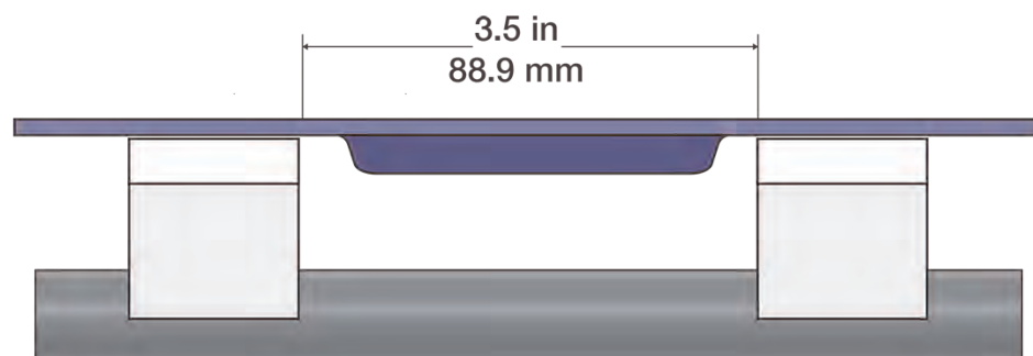
Figura 77: Fila di denti singola tra le guide di contenimento
