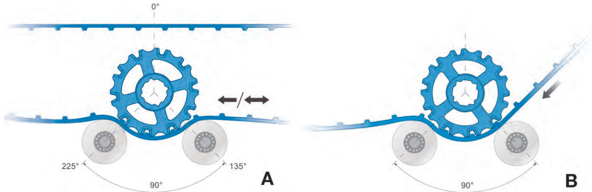
Figura 58: Posizione dei limitatori a rullo con azionamento centrale bidirezionale e unidirezionale
