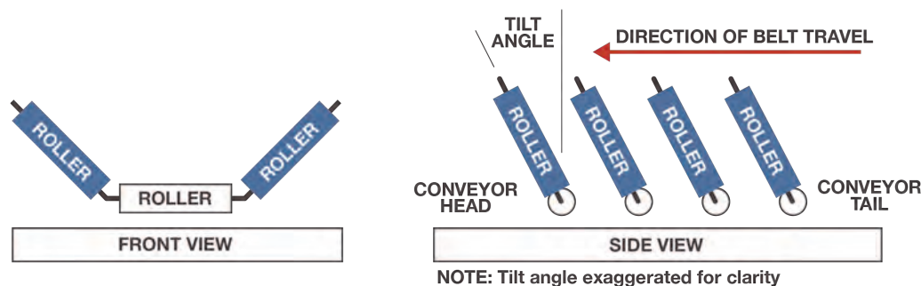
Figura 69: Angoli di inclinazione e direzione di scorrimento del nastro
