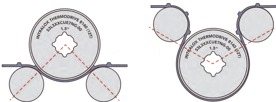
Figura 74: Innesto del nastro-pignone a 90 gradi e 225 gradi
