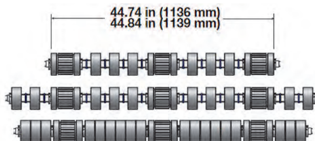
Figura 8: Rulli/distanziali/pignoni a corsia tripla S8240
