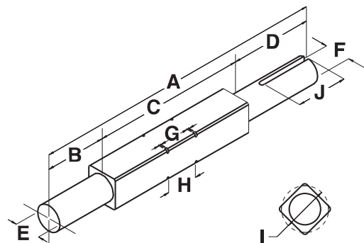
Figura 15: Componenti dell'albero
