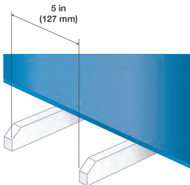
Figura 79: Allineamento delle file di denti nello spazio tra le guide di contenimento
