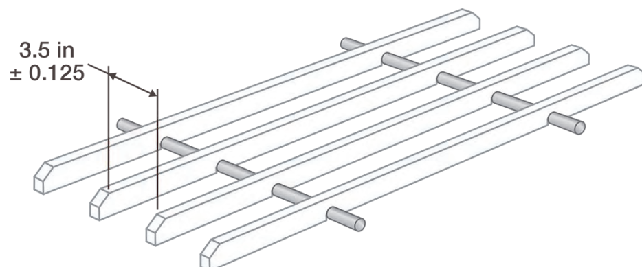
Figura 78: Dimensioni del gioco tra le guide di contenimento
