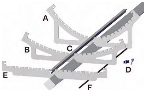
Figura 21: Componenti del convertitore con configurazione a conca
