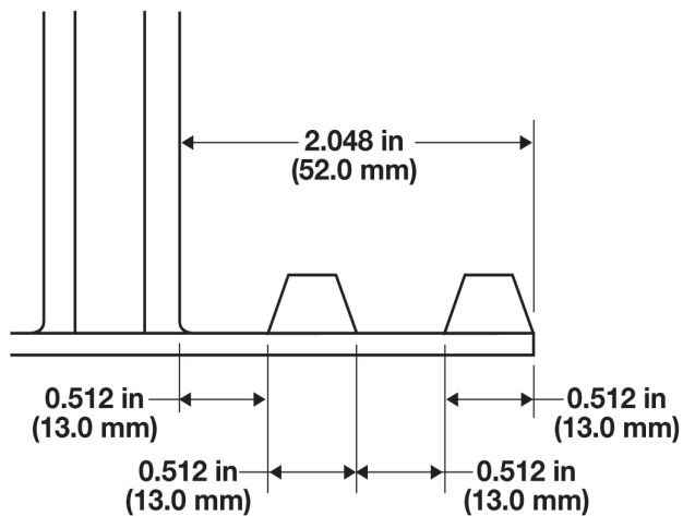
Figura 13: Margini per due corsie della guida trapezoidale
