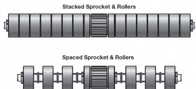
Figura 6: Rulli/distanziali/pignoni a corsia singola S8240
