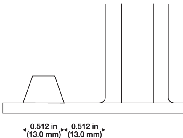
Figura 12: Margini per una corsia della guida trapezoidale
