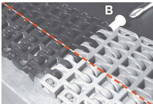
Figure 142: Push rod past older module edge
