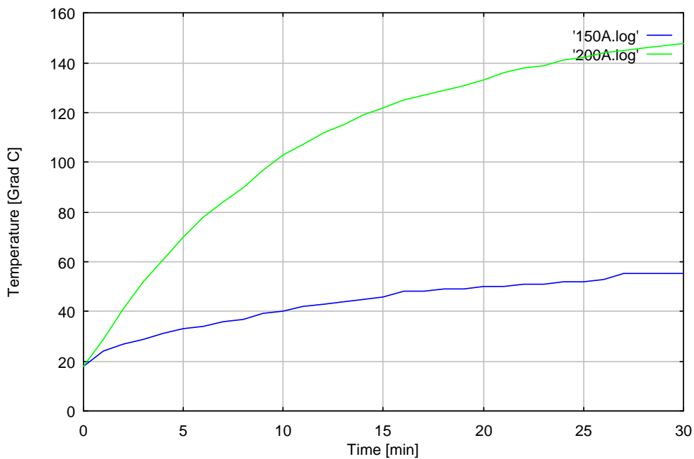
Abb.9: Erwärmungskurven bei Dauerstrombelastung Fig. 9: Heat Up Characteristics at continuous Current
