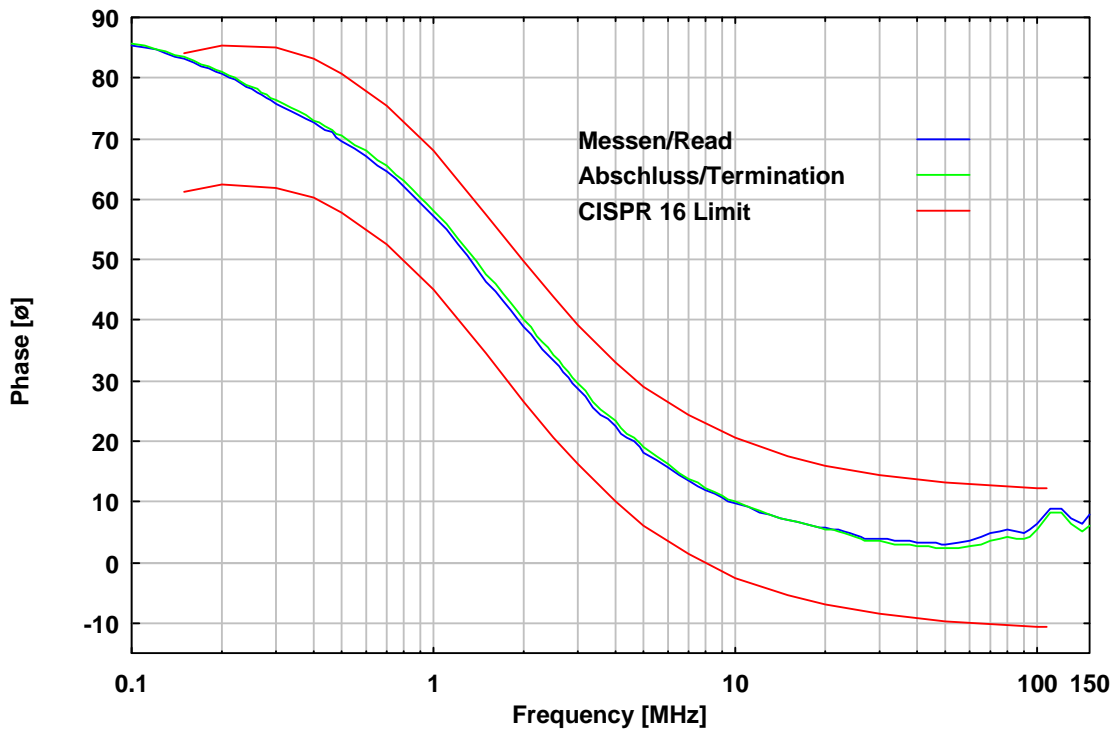
Abb. 5: Phase der Impedanz an den Prüflingsklemmen (Kalibrieradapter KA 8125 erforderlich), BNC mit 50 \Omega Abschluss, Speiseklemmen kurzgeschlossen Fig. 5: Phase of impedance at EuT-Terminals (Calibration adapter KA 8125 required), BNC-Port terminated with 50 \Omega , Mains terminals shorted
