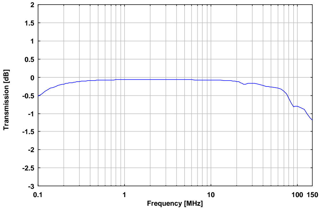
Abb. 7: Spannungsteilungsmaß Prüflingsklemmen - BNC (Spezialadapter erforderlich) Fig. 7: Voltage division ratio EuT-Terminals to BNC (Adapter required)
