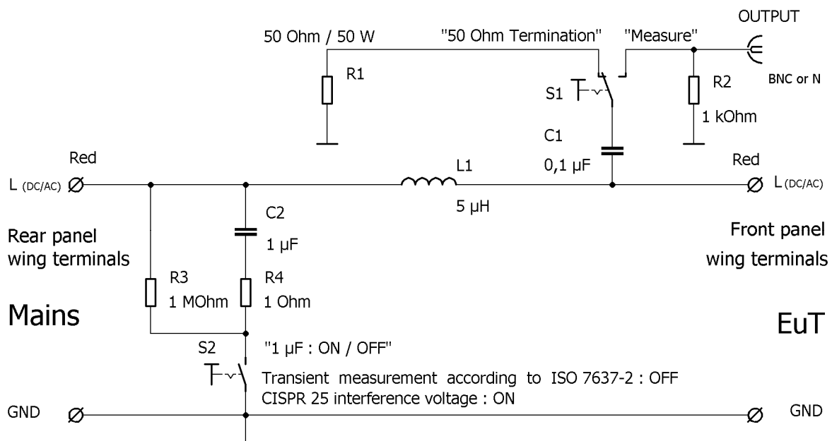
Abb. 2: Prinzipschaltbild NNBM 8124-200 Fig. 2: Schematic circuit diagram of the NNBM 8124-200
