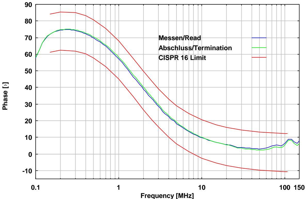
Abb. 6: Phase an den Prüflingsklemmen (Spezialadapter erforderlich), BNC mit 50 \Omega Abschluss, Speiseklemmen offen Fig. 6: Phase at EuT-terminals (adapter required), BNC-port is terminated with 50 \Omega , mains terminals open
