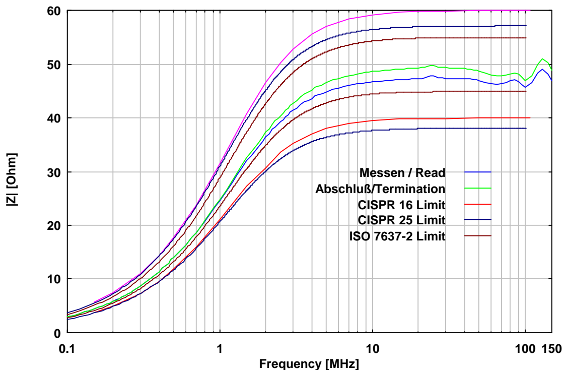
Abb. 4: Betrag der Impedanz an den Prüflingsklemmen (Kalibrieradapter KA 8125 erforderlich), BNC mit 50 Ω Abschluss, Speiseklemmen kurzgeschlossen
