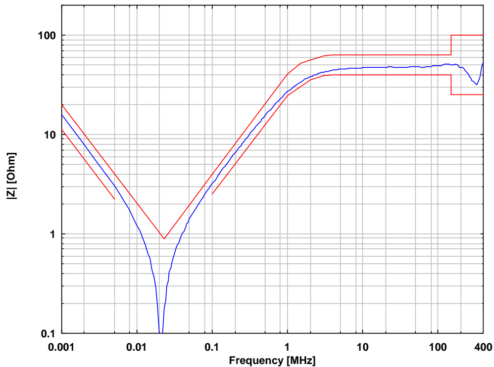
Abb. 9: Betrag der Impedanz an den Prüflingsklemmen nach DEF STAN 59-411 (Kalibrieradapter KA 8125 erforderlich), BNC mit 50 Ω Abschluss, 10 µF Kondensator an den Speiseklemmen Fig. 9: Magnitude of impedance at EuT-Terminals in acc. to DEF STAN 59-411 (Calibration adapter KA 8125 required), BNC-Port terminated with 50 Ω, 10 µF Capacitor across mains terminals
