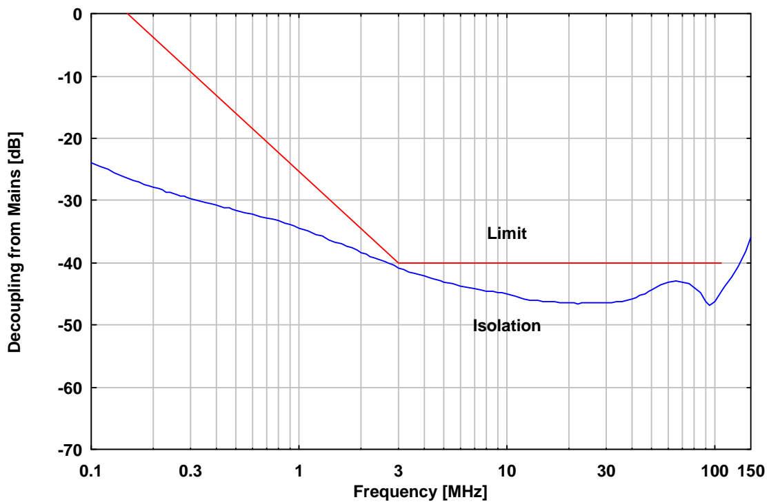
Abb. 8: Entkopplung vom Speisernetz Fig. 8: Decoupling (Isolation) from mains
