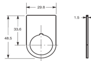
30 x 50 mm Plaque signalétique monopiece
