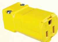
15A, 125V, 2P, 3 wires. # HUBHBL5969VY
