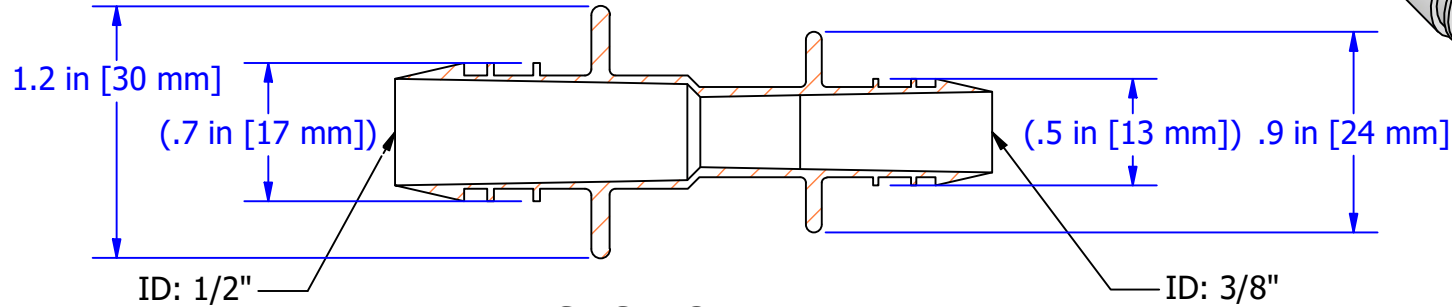
SECTION A-A SCALE 1 : 0.9
