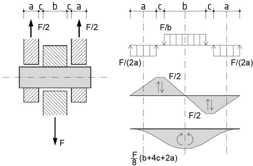
EN - analytical model
