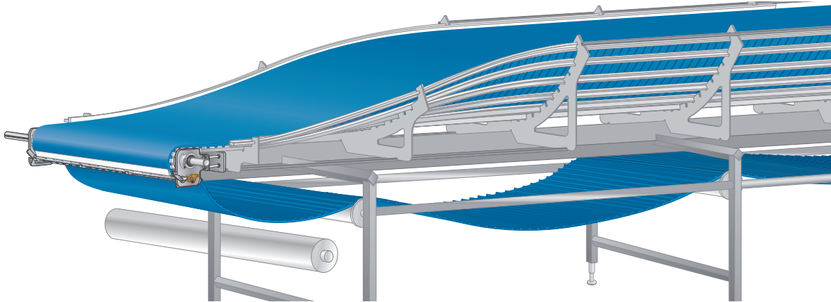
図 19: トラフコンバータ
