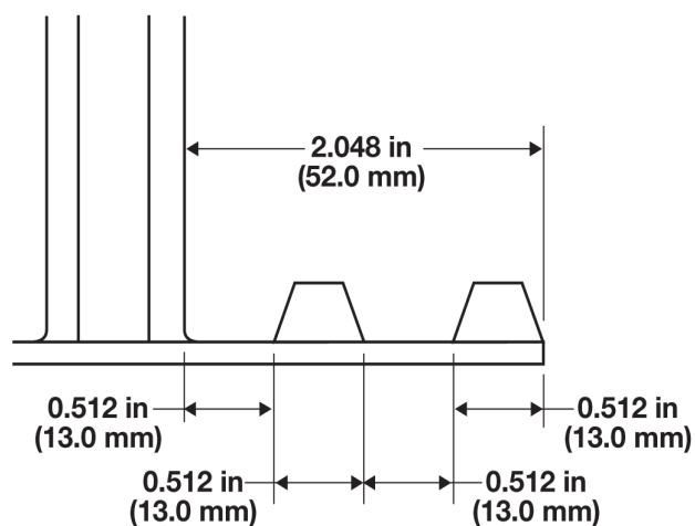
図 10: V ガイド 2 レーン分のインデント
