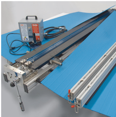
図 21: ThermoDrive®ストリームライン接合セットとコンポーネント
