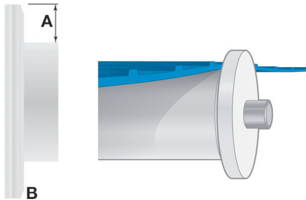
図 62: 最小クリアランスと必要な面取り
