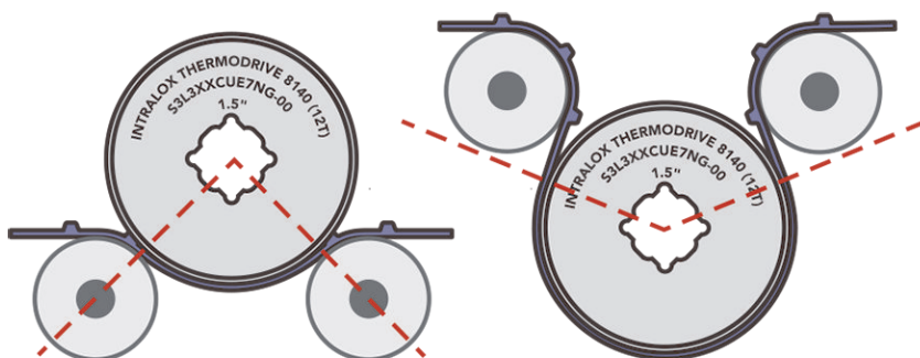
図 72: 90 度および 225 度のベルトとスプロケットの噛み合い
