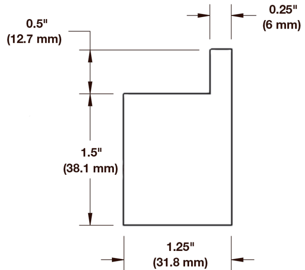
図 18: フランジ付きウェアストリップの寸法
