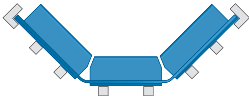
図 84: U 形ベルト上面走行路（キャリア側）
