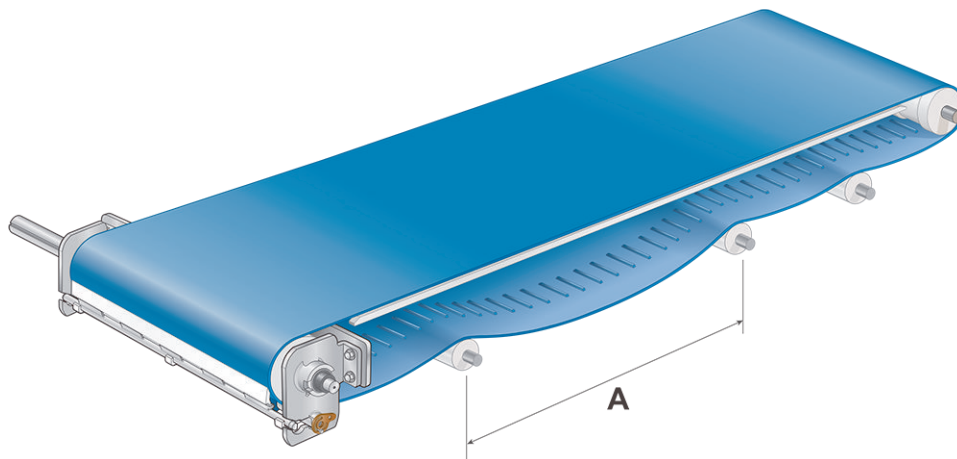
図 69: 正しいサポートの間隔
