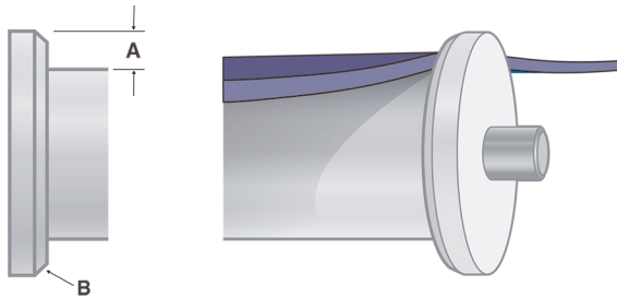
図 79: 必要な最低高さと同面取り
