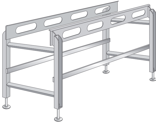
図 28: 衛生処理のためにたやすくアクセスできる簡単な構造
