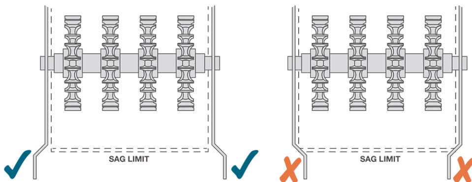
図 40: 適切なクリアランス
