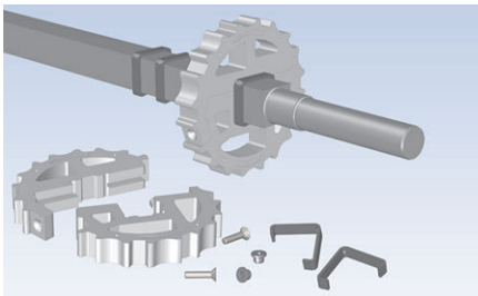
図 14: セルフセット固定リング
