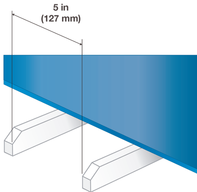
図 77: 保持レール間の隙間内のラグの配置
