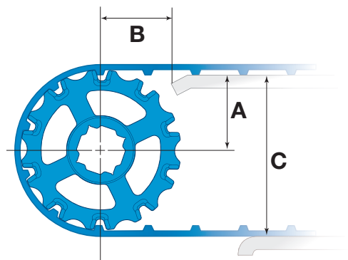
図 11: 駆動側寸法
