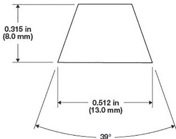
図 8: V ガイドの公称形状
