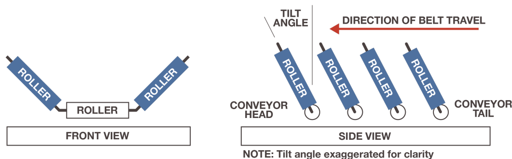
図 67: ベルト進行方向と傾斜角
