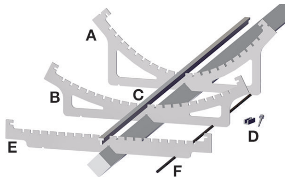
図 20: トラフコンバータのコンポーネント
