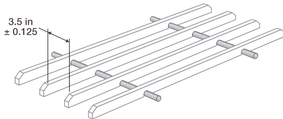
図 76: 保持レール間の隙間の寸法
