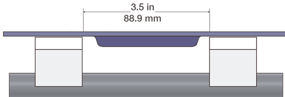
図 75: 保持レール間のシングルラグ
