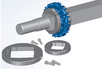
図 13: 分割重荷重用固定リング
