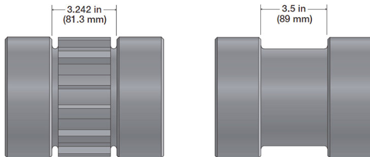
図 74: スプロケットとローラー内側寸法
