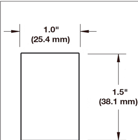
図 17: フラットウェアストリップの寸法
