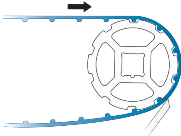
図 57: 斜めに取り付けたスクレイパー
