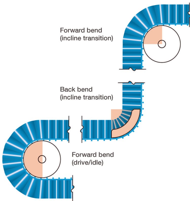
図 6: 高巻き付き角（以下の S8050 同期サイドウォールのデータ表を参照）
