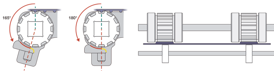
図 73: ポジションリミターの 165°~180°での配置
