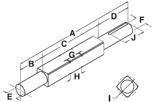
図 12: シャフトコンポーネント
