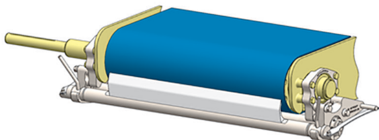
図 16: TD 駆動装置（先頭駆動）
