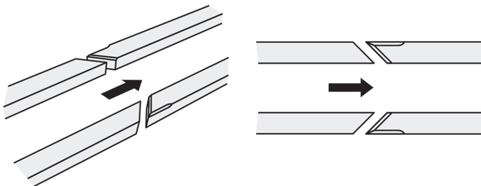
図 66: 45°角に面取りされたレール
