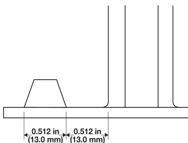
図 9: V ガイド 1 レーン分のインデント
