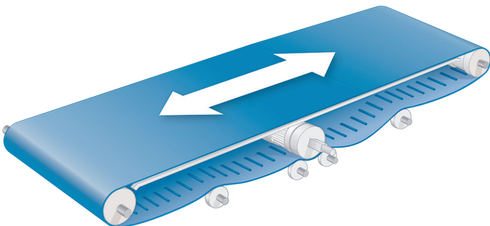
図 71: センター駆動sprocketとポジションリミターの位置
