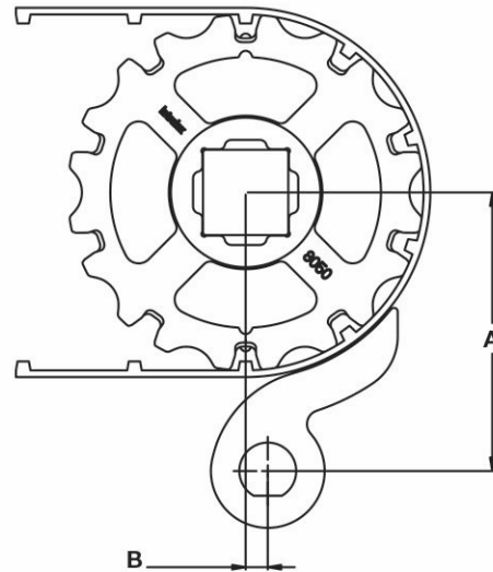
S8026 ポジションリミター (ユニバーサルマウント) の設置寸法
