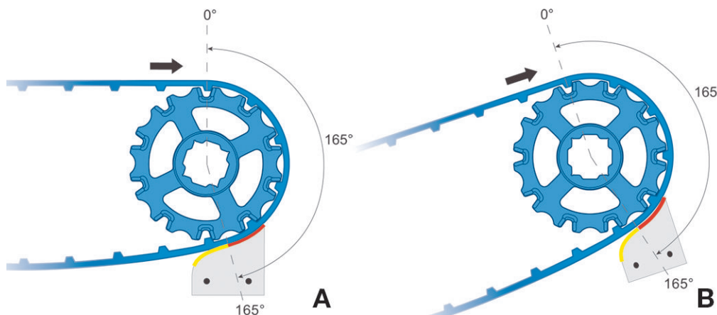
図 54: 先頭駆動のポジションリミターの配置
