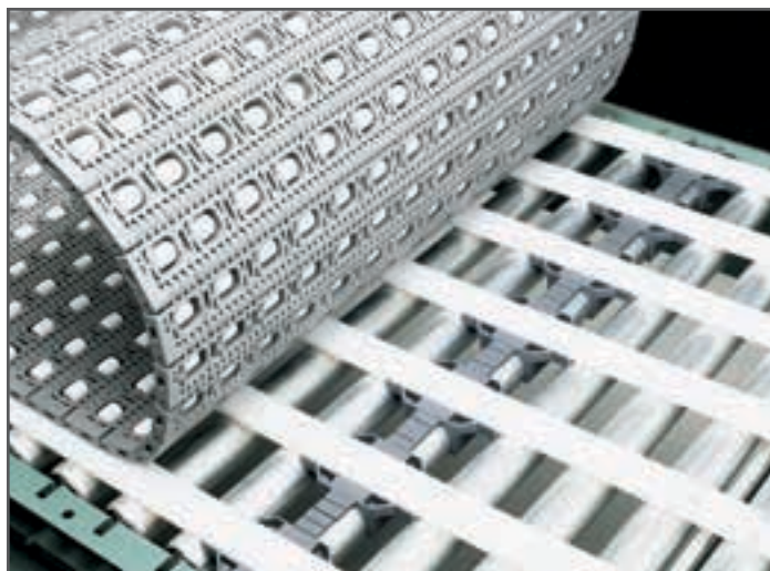
S400 Roller Top Retrofit è facile da installare sui trasportatori a rullo esistenti, risparmiandovi elevati costi di sostituzione.
