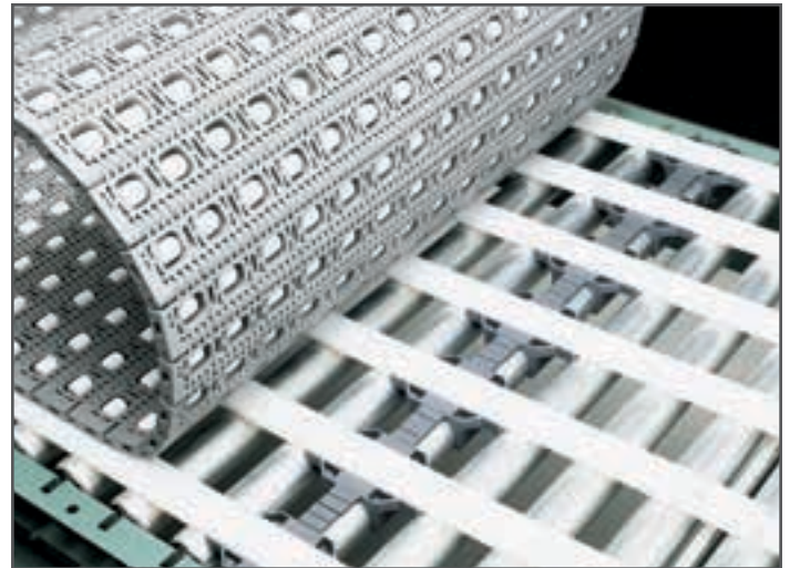
Le système S400 Roller Top Retrofit est facile à installer sur des convoyeurs à rouleaux existants, ce qui permet d'éviter des coûts de remplacement onéreux.
