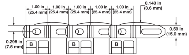
Şekil 76: S2700 Side Drive 2.0
