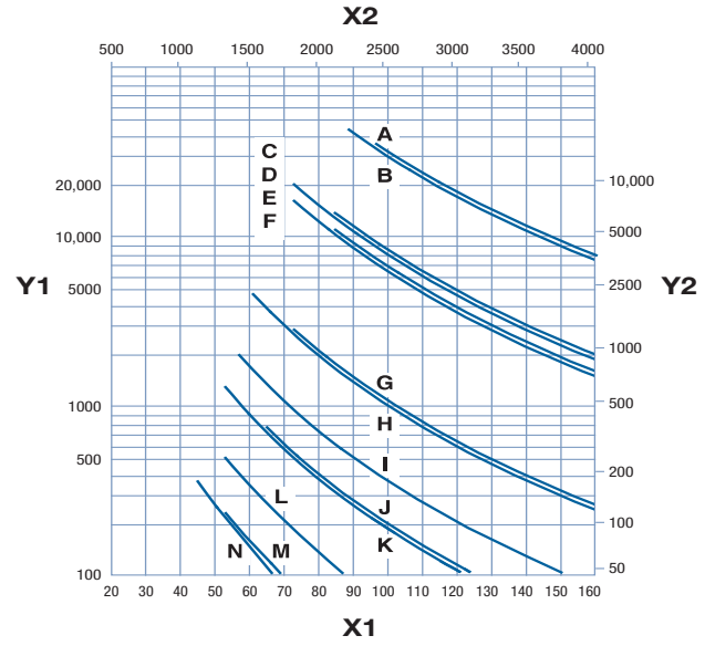
Şekil 192: Üç (3) veya daha fazla eşit aralıklı rulmanlı çift yönlü ve itici konveyörler; izin verilen maksimum defleksiyon: 0,22 inç (5,6 mm)
