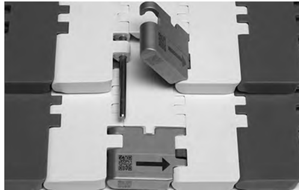
Şekil 14: Temiz Ayırma modeli
