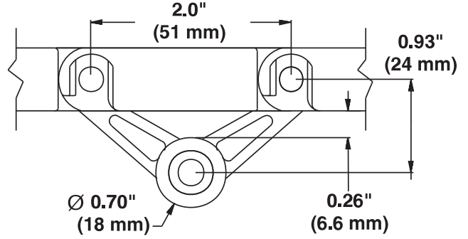
Şekil 114: Geri tutma ruloları, yandan görünüm
