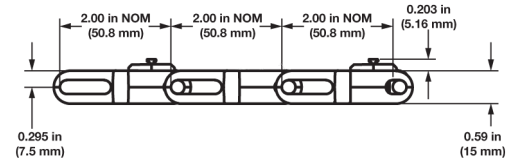
Şekil 80: Mini Rib yerleştirme elemanlı modül
