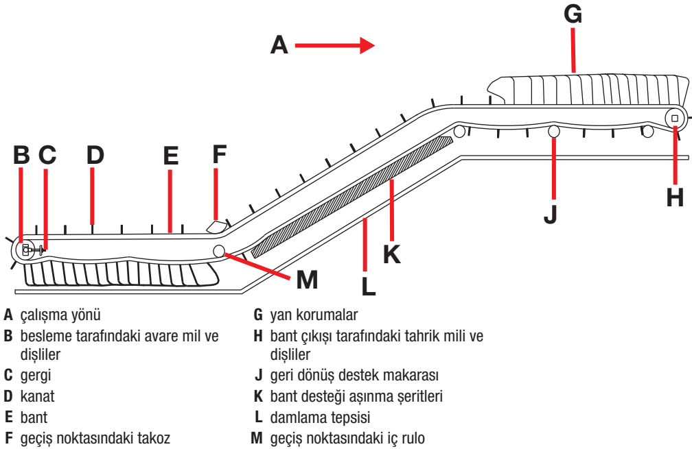
Şekil 162: Üç kısımlı yukarı/aşağı eğimli konveyör
