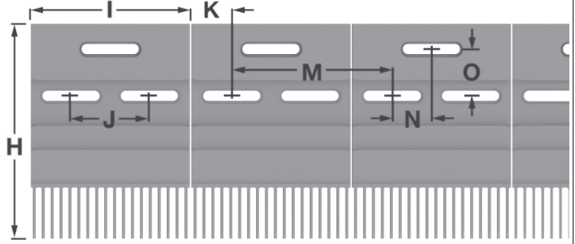
S400 Kendi Temizlenen Taraklı Transfer Plakası Montajı için Ölçü Gereklilikleri a
