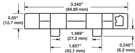
Şekil 44: S1400 Mold to Width Flat Top 85 mm
