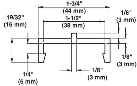
Şekil 103: Çengelli ayaklı takmalı UHMW aşınma şeritleri (B6XX24IXXWMV)
