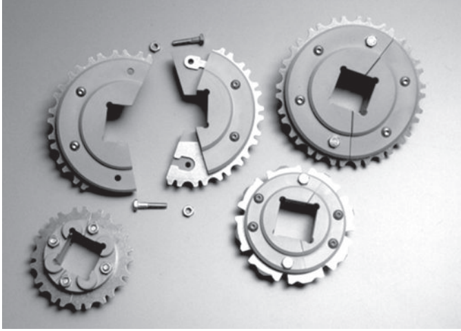
Şekil 115: Parça dişliler
