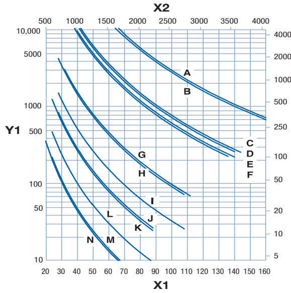
Şekil 189: Yalnızca iki (2) rulmanlı konvansiyonel konveyörler; izin verilen maksimum defleksiyon: 0,10 inç (2,5 mm)
