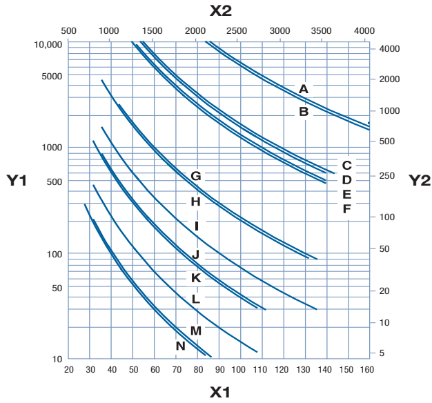
Şekil 191: Yalnızca iki (2) rulmanlı çift yönlü ve itici konveyörler; izin verilen maksimum defleksiyon: 0,22 inç (5,6 mm)
