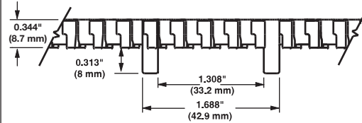
Şekil 25: Seri 900 Flush Grid Mold to Width
