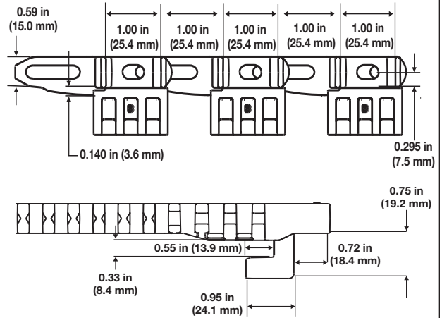
Şekil 78: S2700 Side Drive V2 2.0
