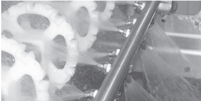
Şekil 112: Püskürtme yapısı, bandın alt tarafının, dişlilerin ve milin temizliğini sağlayacak şekilde tasarlanmıştır
