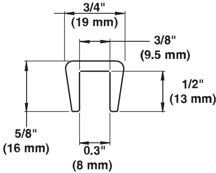
Şekil 104: Standart çubuk oturtmalı UHMW aşınma şeritleri (B6XX28IXXWMV)
