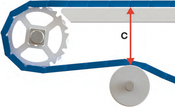
Şekil 124: C tahrik boyutu
