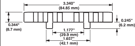
Şekil 26: Seri 900 Flush Grid 85 mm Mold to Width
