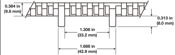
Şekil 30: S900 Flat Top Mold to Width
