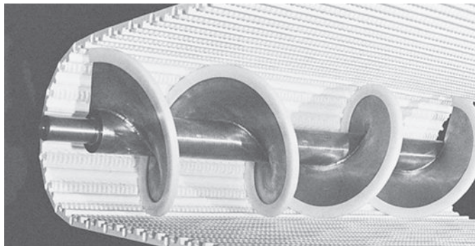
Şekil 94: Avare merdanesi
