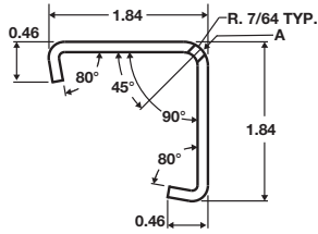
Şekil 88: Kendinden ayarlı tutma bileziği boyutları
