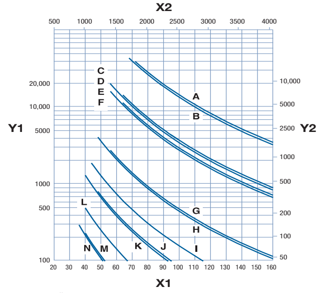
Şekil 190: Üç (3) veya daha fazla eşit aralıklı rulmanlı konvansiyonel konveyörler; izin verilen maksimum defleksiyon: 0,10 inç (2,5 mm)
