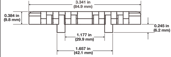
Şekil 31: S900 Flat Top 85 mm Mold to Width
