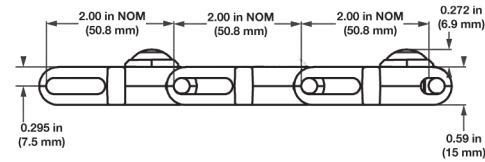
Şekil 79: Friction Top yerleştirme elemanlı modül
