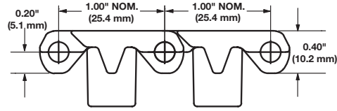
Şekil 49: Yandan görünüm
