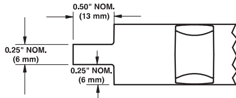
Şekil 61: Seri 2200 tab edge boyutları
