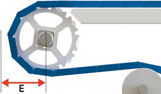
Şekil 126: E tahrik boyutu
