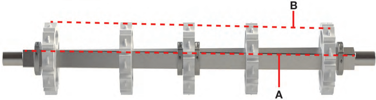
Şekil 151: Mil burulması
