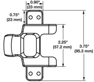
Düz ve dönüşlü versiyonlar için uzatılmış çıkıntılar
