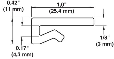
Şekil 99: Takmalı UHMW aşınma şeritleri (B6XX25IXXWMV)
