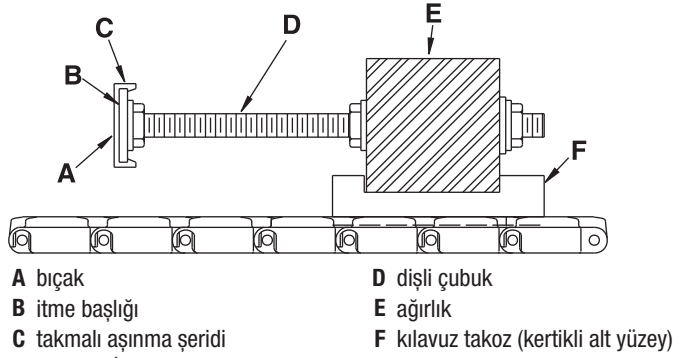
Şekil 108: İtme kolu kurma
