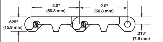
Şekil 17: Polietilen bantlar
