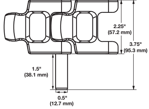
Düz ve dönüşlü versiyonlar için uzatılmış pimler
