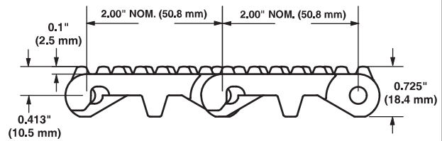
A İç resim: polietilen kenar modülü
