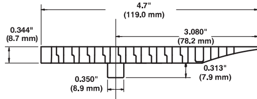
Şekil 28: 4,7 inç (119 mm) tek kılavuz askılı bant
