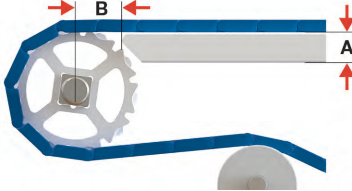
Şekil 123: B tahrik boyutu
