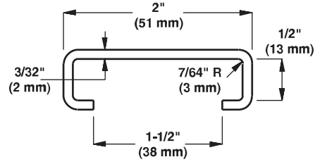
Şekil 101: Kılavuz rayı oturtmalı UHMW aşınma şeritleri (B6XX27IXXWMV)
