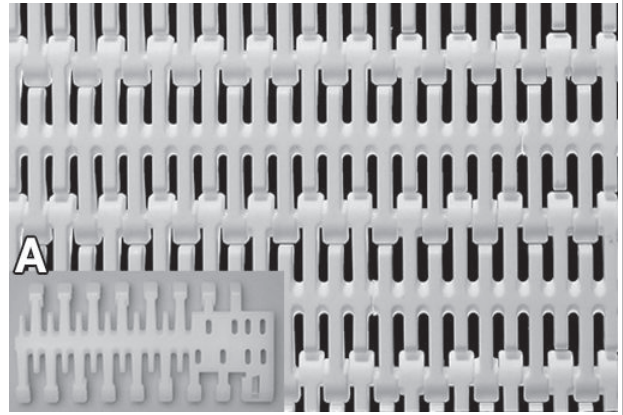
A iç resim: polietilen kenar modülü
