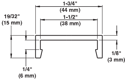
Şekil 102: Çengelli takmalı UHMW aşınma şeritleri (B6XX23IXXWMV)
