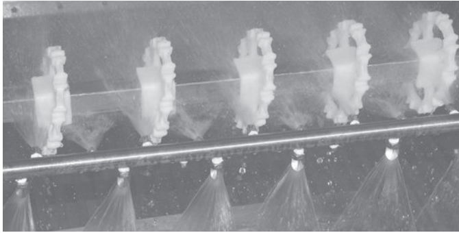
Şekil 111: EZ Clean In Place (CIP) Sistemi
