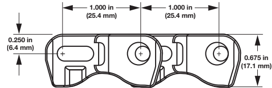
Şekil 66: Düz kenar boyutları
