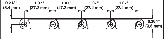
Şekil 36: Boyutlar
