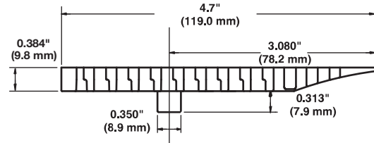
Şekil 33: 4,7 inç (119 mm) tek kılavuz askılı bant
