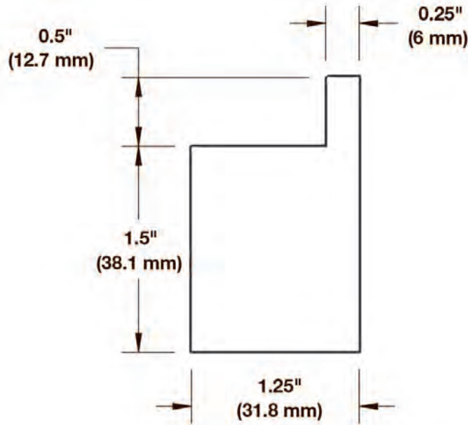
Şekil 97: Flanşlı aşınma şeridi boyutları
