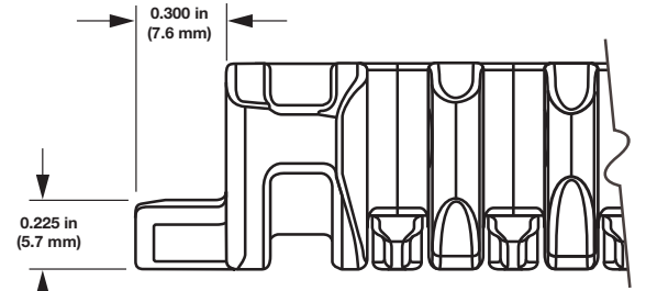
Şekil 65: Askı kenar boyutları
