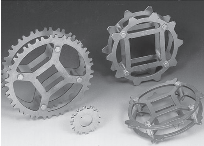
Şekil 116: Aşınmaya dirençli (tamamen çelik) dişliler
