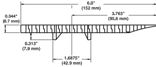
Şekil 27: 6,0 inç (152 mm) çift kılavuz askılı bant
