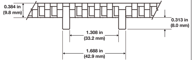
Şekil 37: S900 Flat Top 4,5 inç Mold to Width
