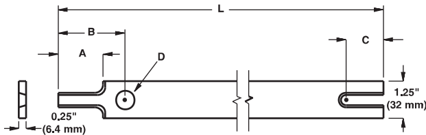
Şekil 95: İç içe geçmeli ek aşınma şeritleri
