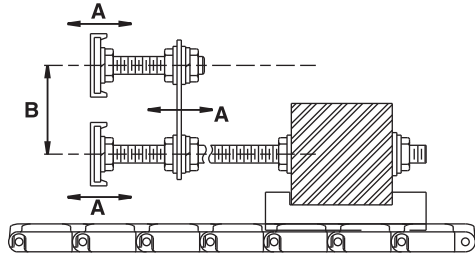
Şekil 109: Çift bıçaklı itme kolu kurma
