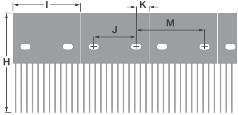
S100 Taraklı Transfer Plakası Montajı için Ölçü Gereklilikleri
