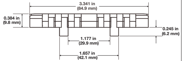
Şekil 38: S900 Flat Top 85 mm Mold to Width
