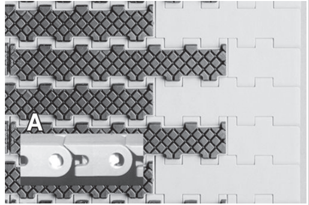
A iç resim: Slidelox çubuk tutma unsuru
