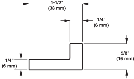
Şekil 98: Standart açılı UHMW aşınma şeritleri (B6XX21IXXWMV)
