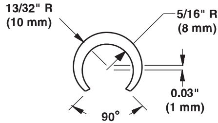
Şekil 105: Tam yuvarlak oturtmalı UHMW aşınma şeritleri (B6XX29IXXWMV)
