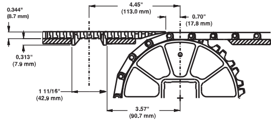
Şekil 29: Kurulum boyutları
