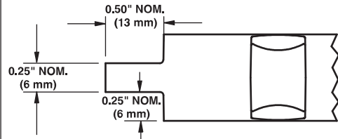
Şekil 62: Askılı kenar boyutları
