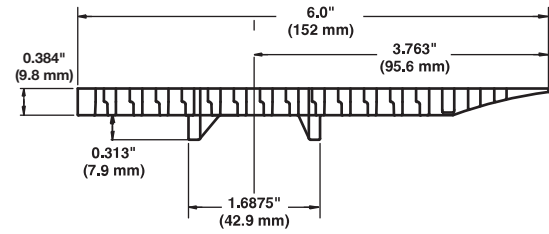
Şekil 32: 6,0 inç (152 mm) çift kılavuz askılı bant
