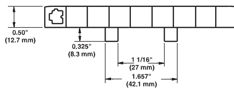
Şekil 43: S1400 Mold to Width Flat Top
