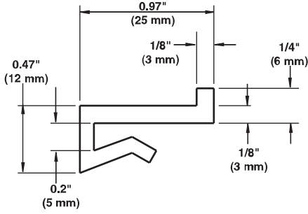
Şekil 100: Ayaklı takmalı UHMW aşınma şeritleri (B6XX26IXXWMV)
