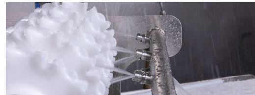
Barra com pulverizador de água para limpeza no local (CIP)
