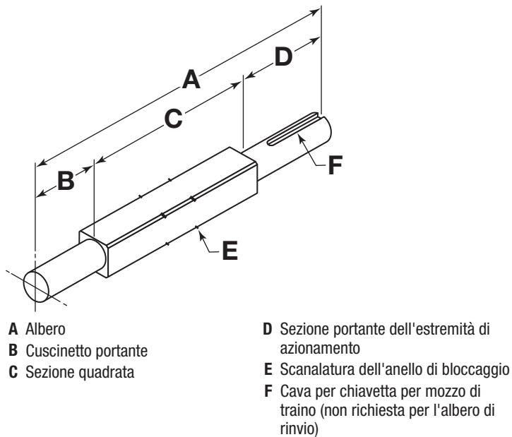
Figura 46: Componenti dell'albero motore a sezione quadrata
