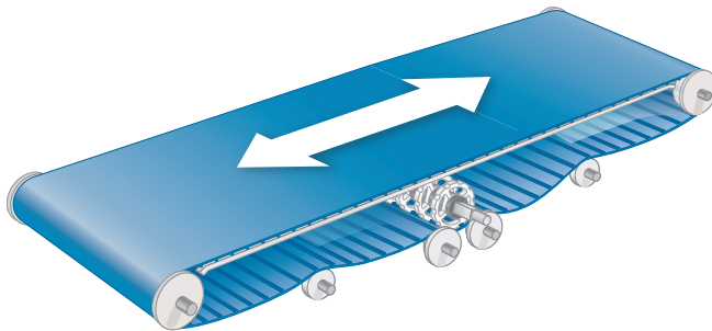
Figura 55: Posizione del pignone di azionamento centrale e del limitatore di posizione
