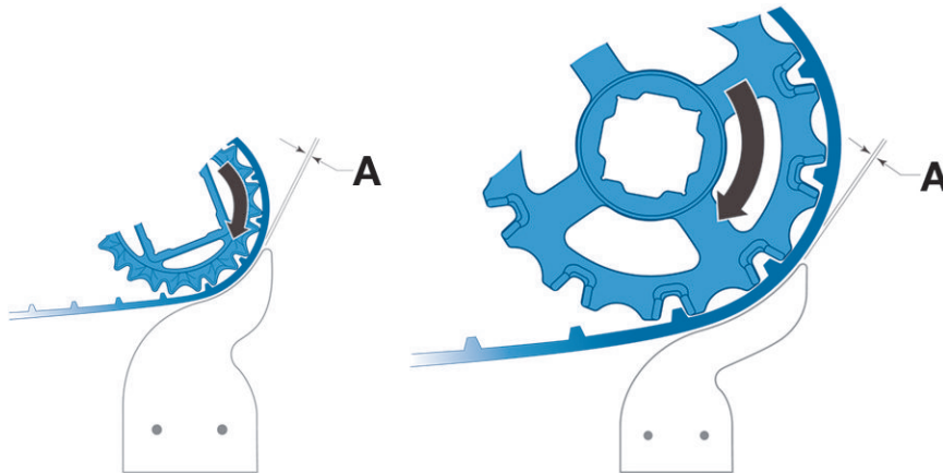
Figura 50: Corretto posizionamento del limitatore
