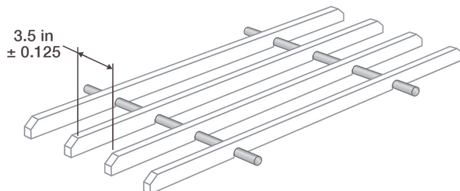
Figura 76: Dimensioni del gioco tra le guide di contenimento
