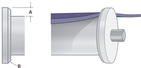
Figura 79: Altezza e smussatura minime richieste
