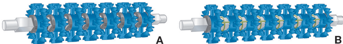
Figura 48: Anelli di bloccaggio e distanziali per pignoni
