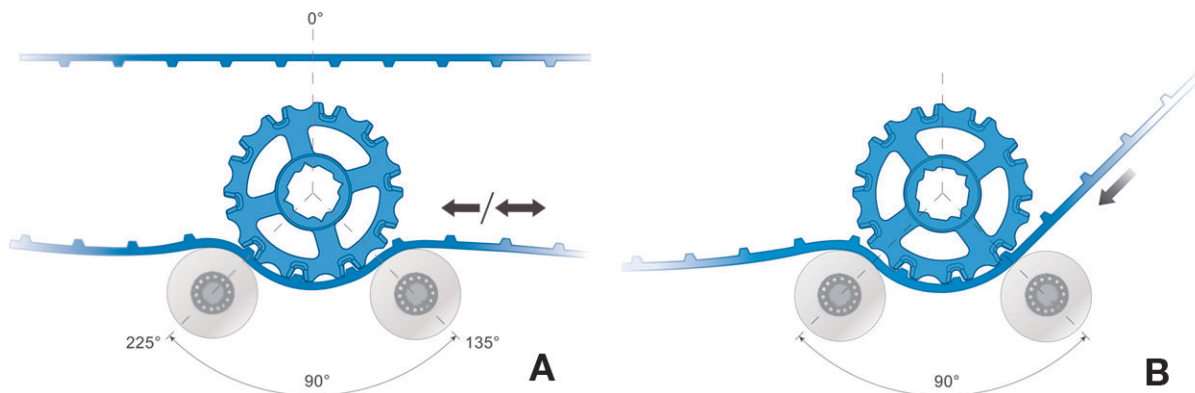
Figura 56: Posizione dei limitatori a rullo con azionamento centrale bidirezionale e unidirezionale
