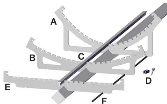
Figura 20: Componenti del convertitore con configurazione a conca
