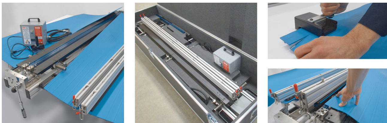
Figura 21: Sistema di giunzione ottimizzato ThermoDrive® e componenti
