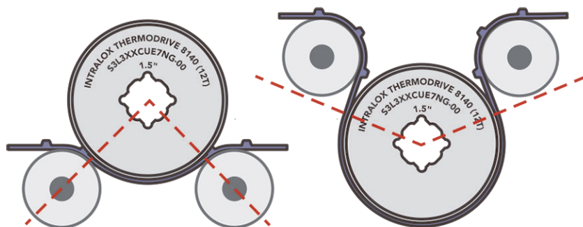
Figura 72: Innesto del nastro-pignone a 90 gradi e 225 gradi
