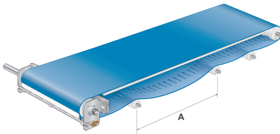
Figura 69: Corretta spaziatura del supporto
