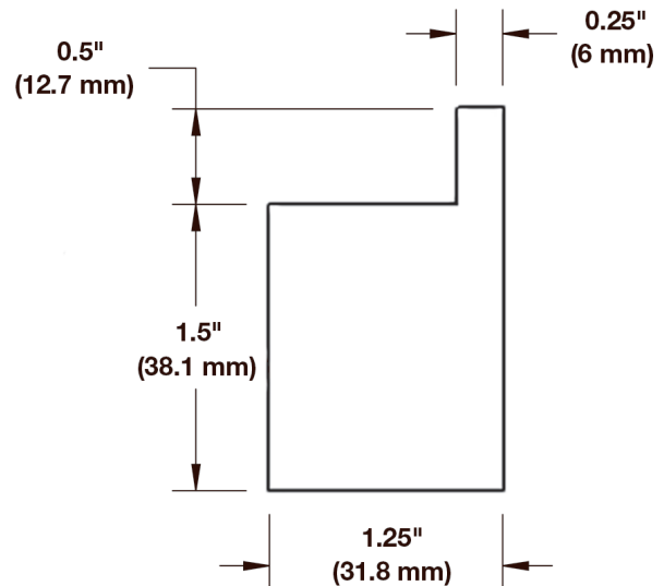
Figura 18: Dimensioni della guida antiusura flangiata
