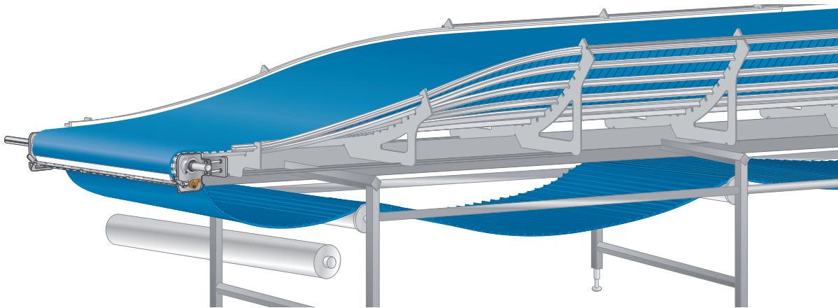
Figura 19: Convertitore con configurazione a conca
