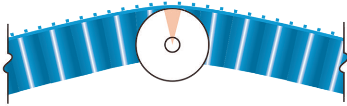
Figura 7: Basso angolo di avvolgimento (vedere la seguente tabella dei dati sulle Synchronized Sidewall S8050)
