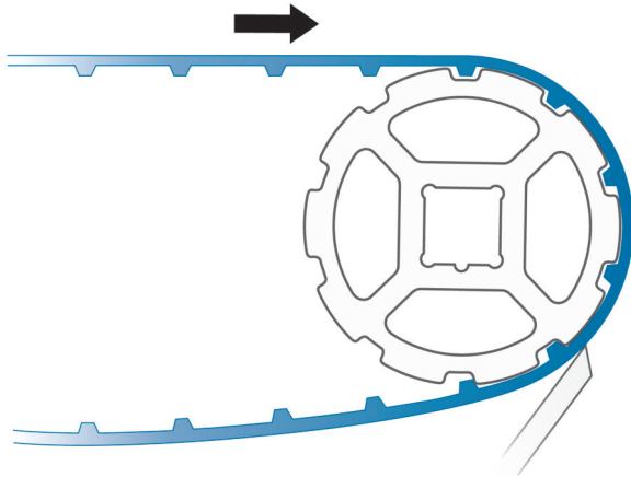
Figura 57: Raschiatore con montaggio in posizione inclinata
