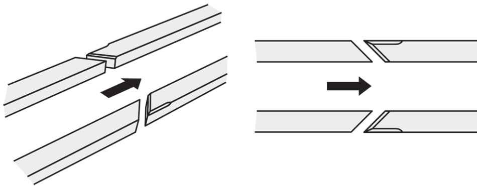
Figura 66: Guide smussate a un angolo di 45°
