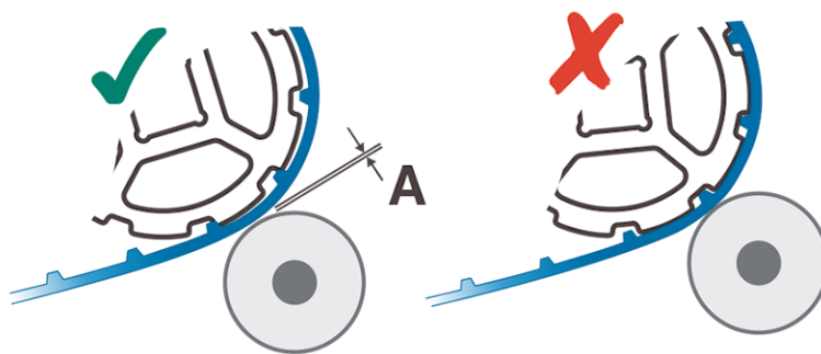
Figura 51: Posizionamento corretto del dente del pignone al di sotto del nastro durante il posizionamento del limitatore a rullo
