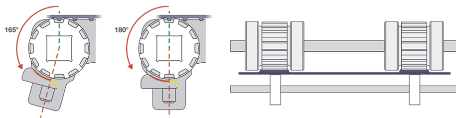
Figura 73: Posizionamento del limitatore di posizione tra 165 e 180 gradi
