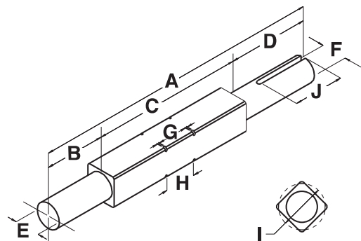
Figura 12: Componenti dell'albero
