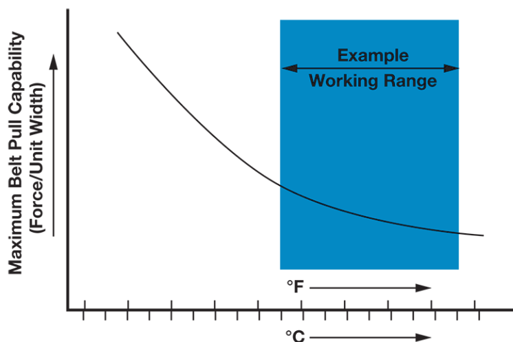
Figura 85: Effetti della temperatura sulla capacità massima di tiro del nastro
