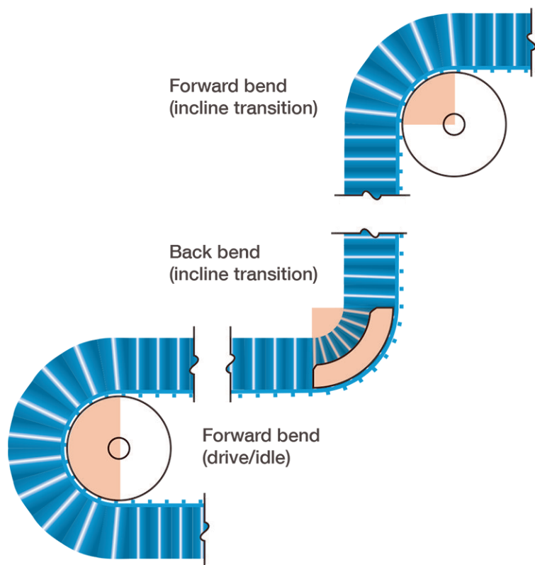
Figura 6: Alto angolo di avvolgimento (vedere la seguente tabella dei dati sulle Synchronized Sidewall S8050)
