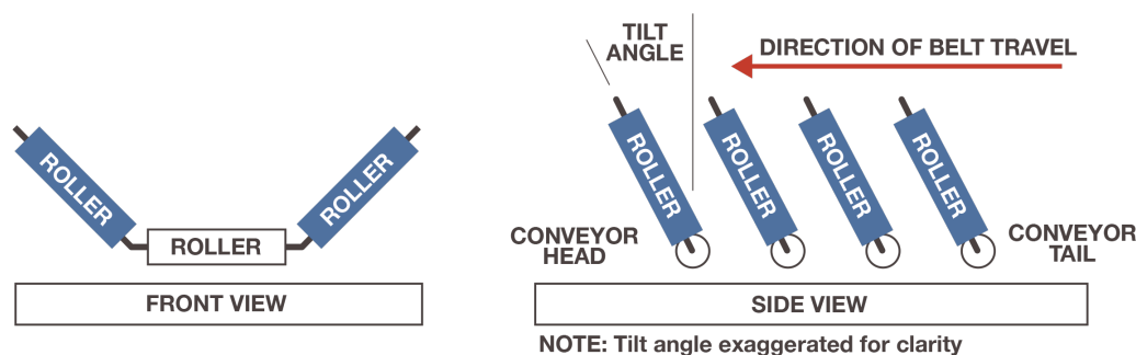
Figura 67: Angoli di inclinazione e direzione di scorrimento del nastro
