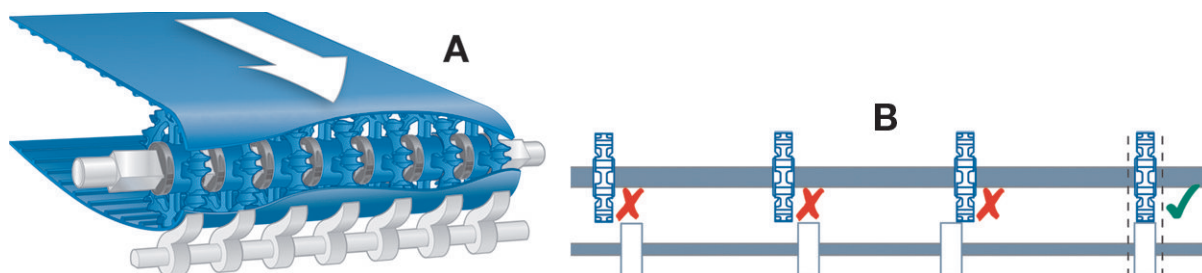
Figura 53: Allineamento e gioco minimo corretti per i nastri senza accessori
