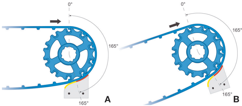
Figura 54: Posizionamento del limitatore di posizione nell'azionamento dall'estremità
