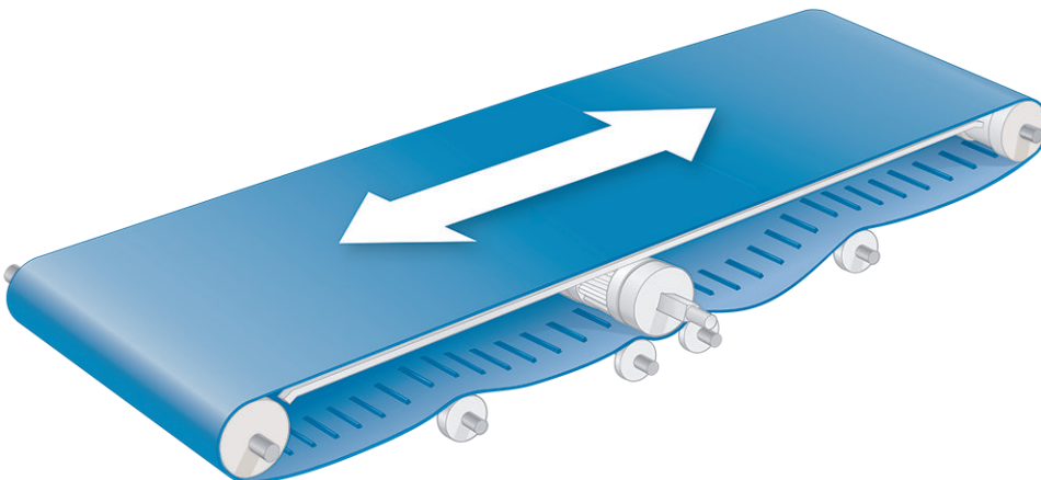
Figura 71: Posizione del pignone di azionamento centrale e del limitatore di posizione
