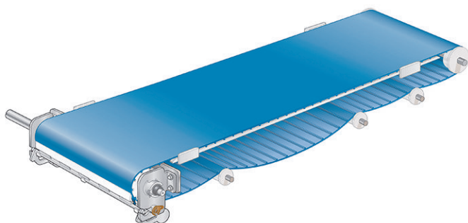
Figura 24: Nastro senza tensionamento
