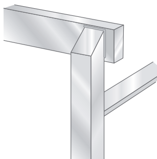
Figura 29: Corretto montaggio dei giunti
