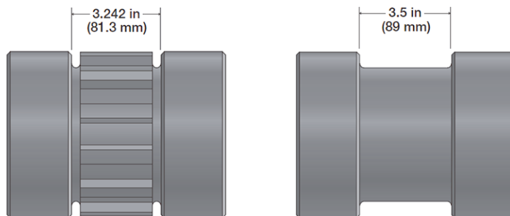
Figura 74: Dimensiones interiores del engranaje y del rodillo
