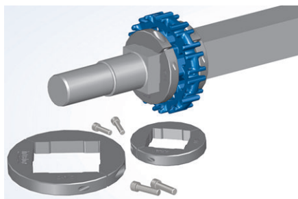
Figura 13: Anillo de retención reforzado bipartido
