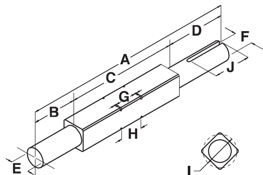
Figura 12: Componentes del eje
