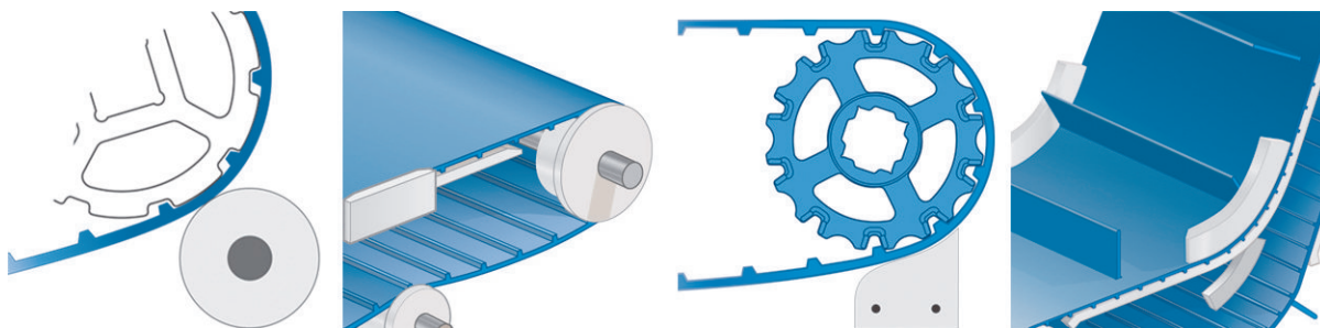
Figura 25: Componentes en el radio de curvatura mínimo o por encima del mismo
