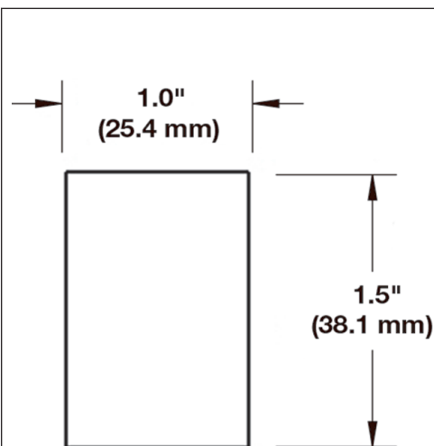
Figura 17: Dimensiones de la guía de desgaste plana
