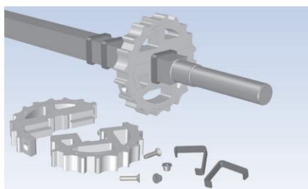
Figura 14: Anillos de retención autoajustables
