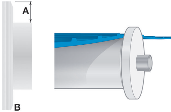
Figura 62: Separación mínima y bisel necesario
