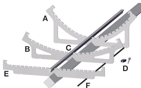
Figura 20: Componentes del transportador de canaleta
