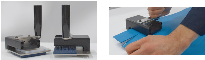
Figura 22: Herramienta de preparación manual de la banda
