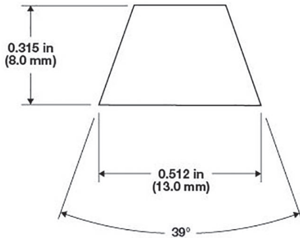
Figura 8: Geometría nominal de la guía en V
