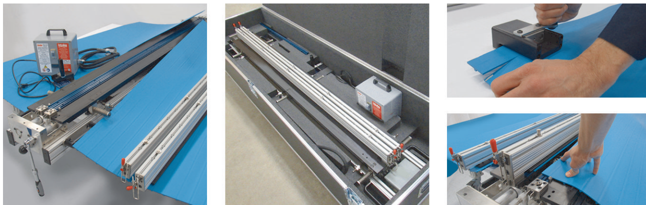
Figura 21: Conjunto de unión térmica optimizado ThermoDrive® y componentes
