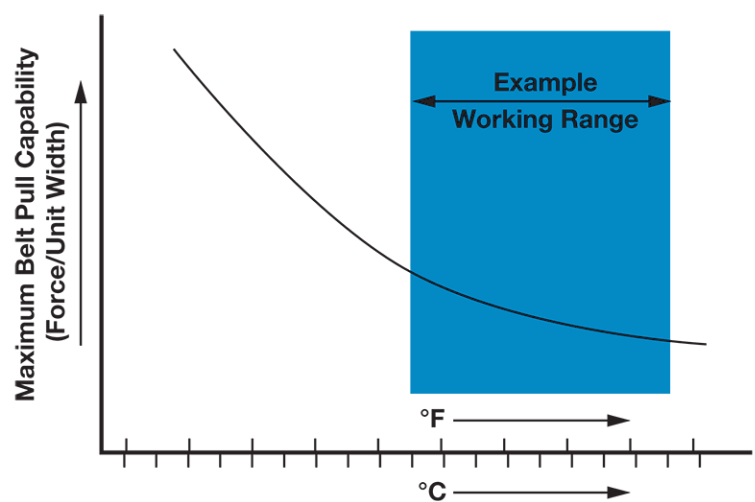
Figura 85: Efectos de la temperatura en la capacidad máxima de tracción de la banda
