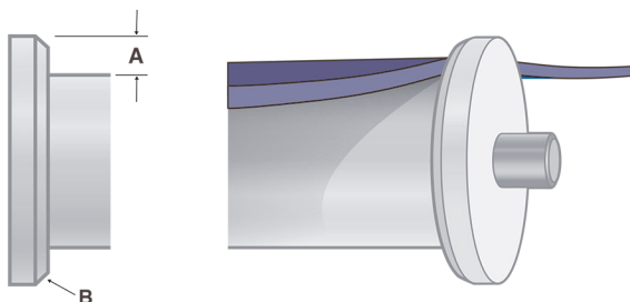
Figura 79: Altura mínima y bisel necesario
