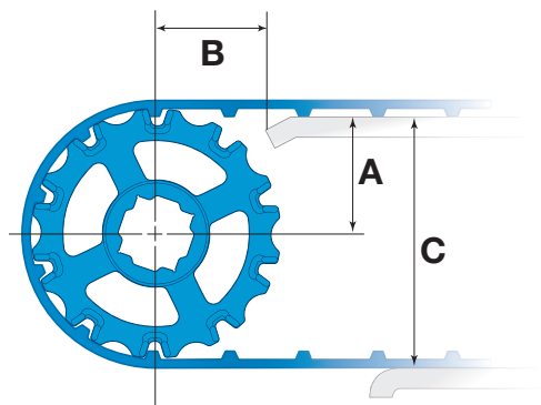
Figura 11: Dimensiones del extremo motriz
