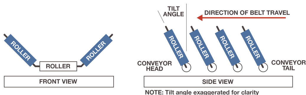
Figura 67: Ángulos de inclinación y dirección de desplazamiento de la banda
