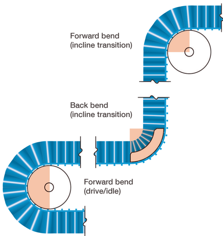
Figura 6: Ángulo de envoltura alto (consulte la siguiente tabla de datos de las paredes laterales sincronizadas S8050)
