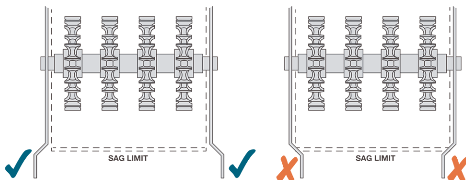
Figura 40: Separación correcta
