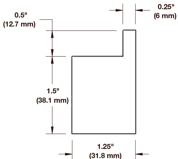
Figura 18: Dimensiones de la guía de desgaste con valona
