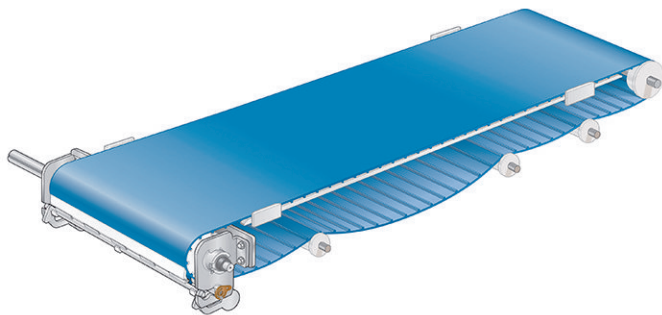
Figura 38: Flexión catenaria entre componentes
