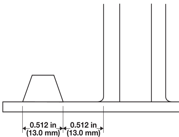
Figura 9: Márgenes laterales para una fila de guía en V
