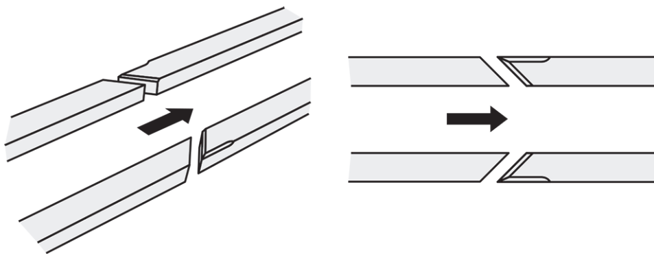
Figura 66: Rieles biselados en un ángulo de 45 grados
