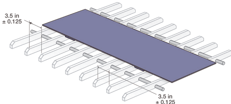
Figura 78: Separación con doble barra de tracción
