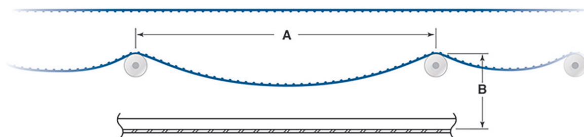
Figura 39: Flexión de catenaria
