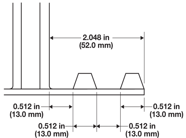
Figura 10: Márgenes laterales para dos filas de guía en V
