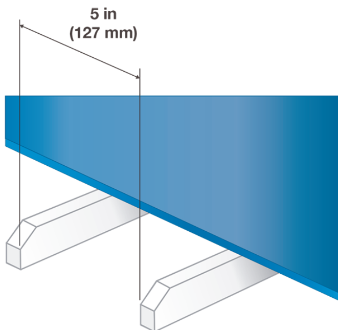
Figura 77: Alineación de la barra de tracción entre los rieles de contención
