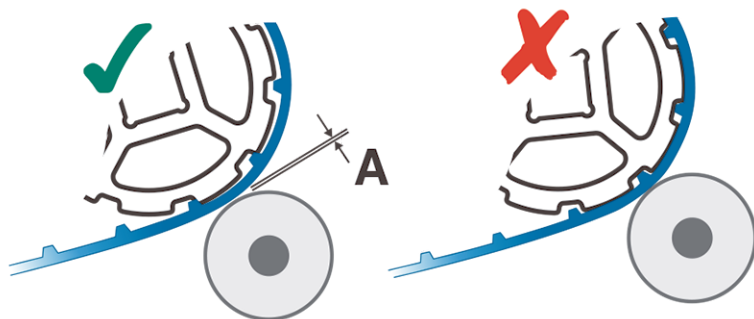
Figura 51: Colocación correcta del diente del engranaje debajo de la banda al colocar el limitador de rodillo
