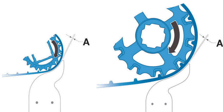
Figura 50: Colocación correcta del limitador
