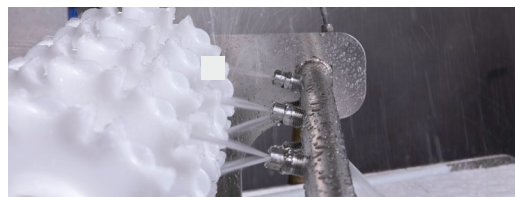
Barre de vaporisation de nettoyage en place (CIP)
